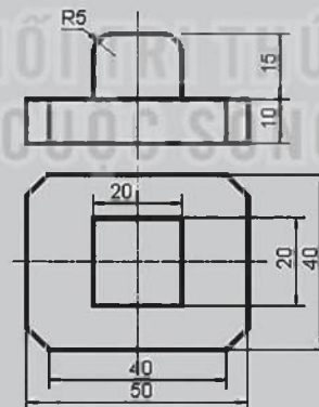
Hình 16.7. Gối đỡ
