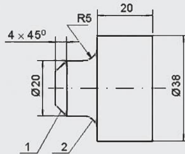
Hình 16.4. Trục
