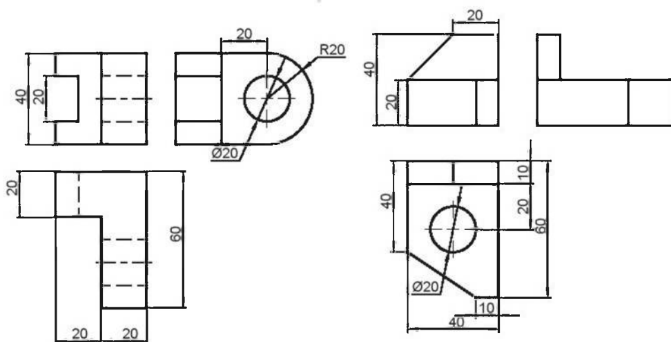
Bản vẽ kỹ thuật giá ngang
