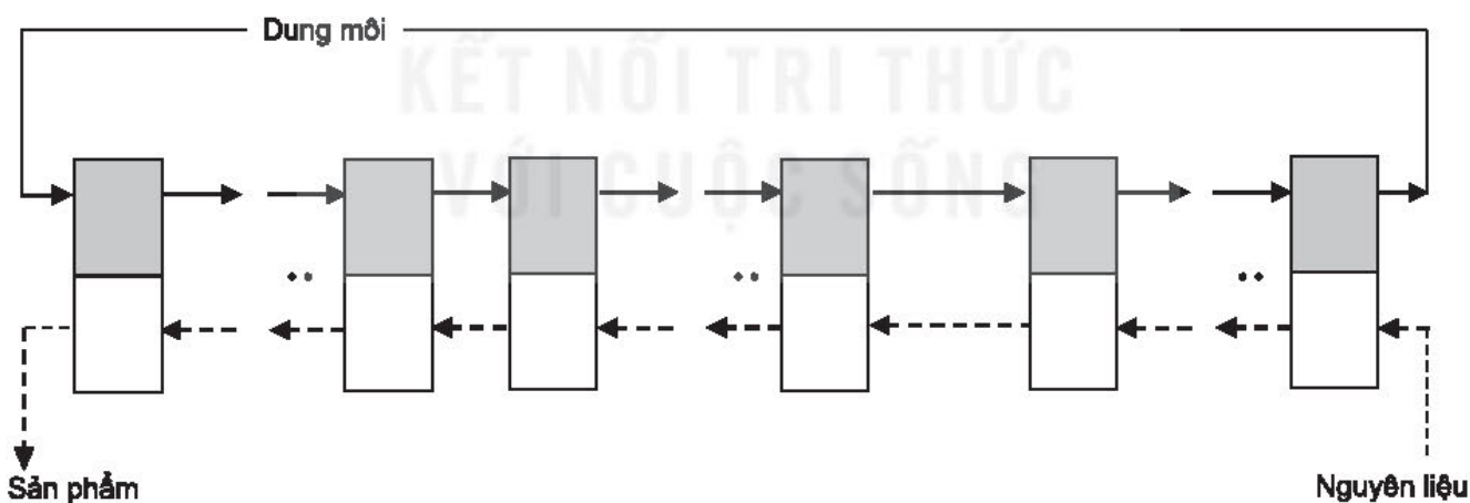
Hình 11.2. Sơ đồ thiết bị chung của quá trình chiết nhiều bậc
