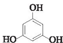
benzene-1,3,5-triol
