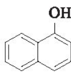
naphthalen-1-ol
