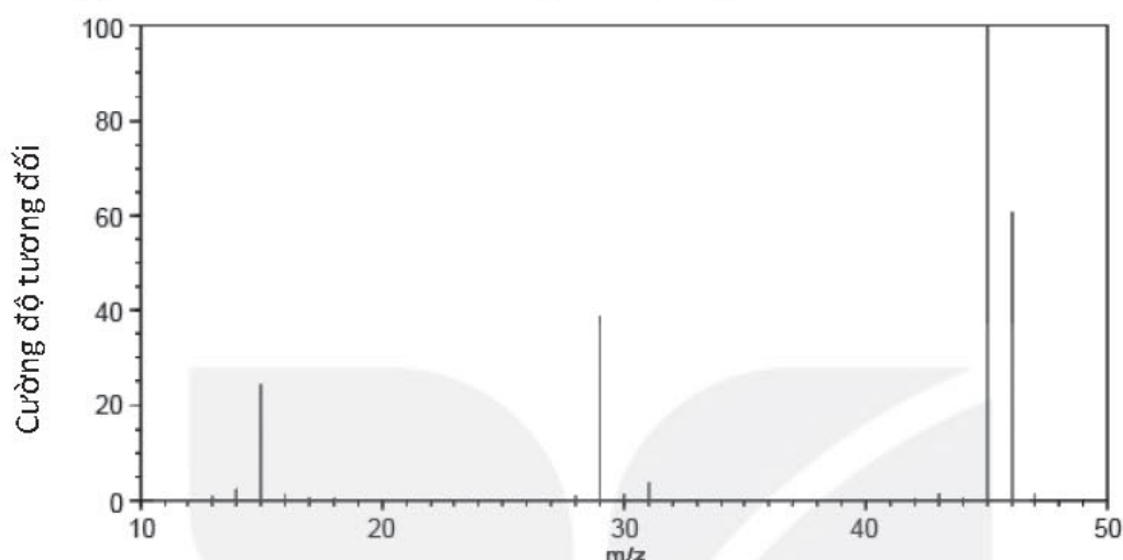
Hình 12.3. Phổ khối lượng của dimethyl ether
