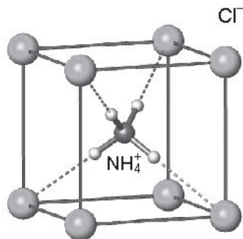
Hình 5.2. Ô cơ sở của \text{NH}_4\text{Cl}
