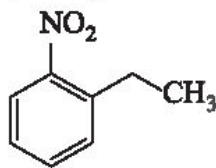
1-ethyl-2-nitrobenzene
