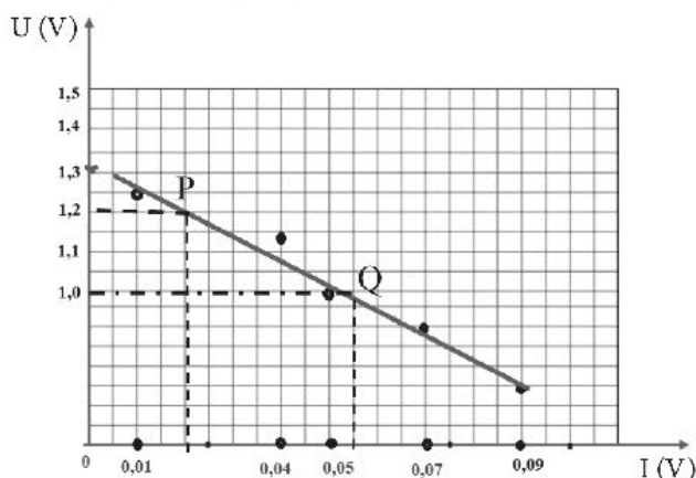
Hình 26.1. Đồ thị quan hệ U và I với pin cũ
