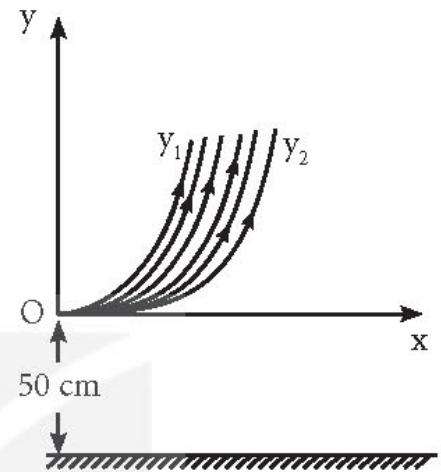
Hình 18.2. Quỹ đạo chuyển động của chùm ion âm
