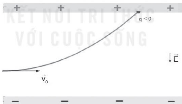
Hình 18.1. Quỹ đạo chuyển động của điện tích âm trong điện trường đều giữa hai bản phẳng nhiễm điện
