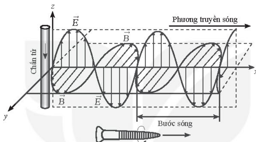
Hình 11.1. Sự lan truyền của sóng điện từ
