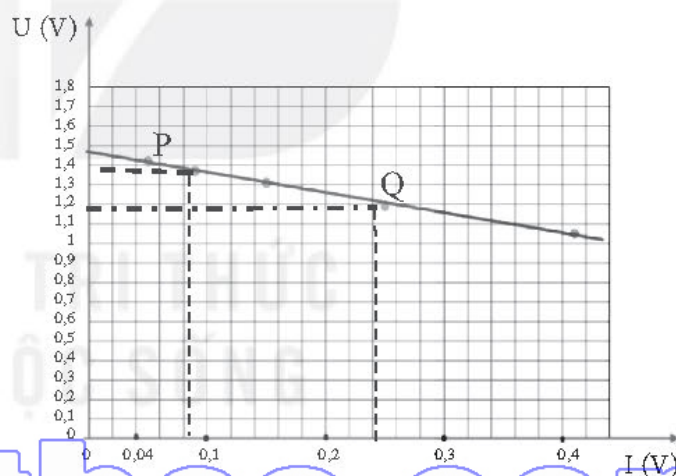
Hình 26.2. Đồ thị quan hệ U và I với pin mới
