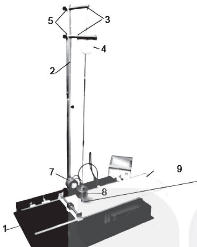
a) Bộ thí nghiệm khảo sát dao động tắt dần của con lắc đơn
