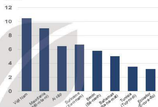
Hình 8.9. Dự báo tác động của hiện tượng dâng mực nước biển 1 m đến GDP (tỷ lệ thiệt hại GDP)
