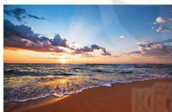
a) Bình minh, Mặt Trời mọc ở hướng Đông
