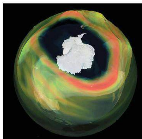
Hình 9.6. Lỗ thủng tầng ozone ở Nam Cực
