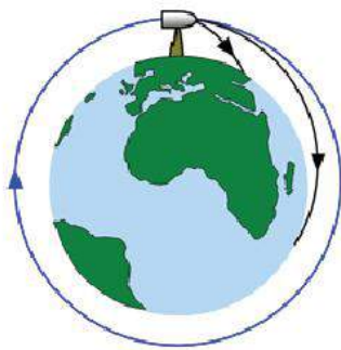
Hình 1.6. Mô hình mô tả ý tưởng phóng viên đạn chuyển động quanh Trái Đất của Newton
