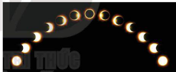
Hình 6.6. Các pha nhật thực
