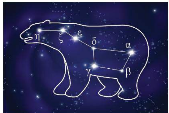
Hình 4.5. Chòm sao Gấu Lớn
