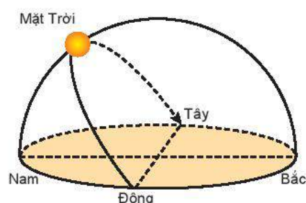
Hình 5.4. Mặt Trời mọc và lặn
