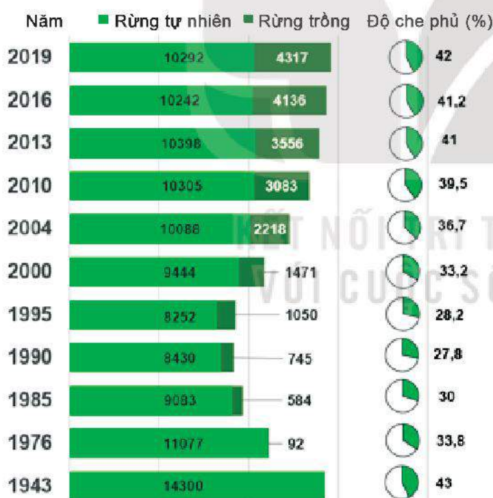
Hình 7.7. Biểu đồ diện tích rừng và độ che phủ rừng ở Việt Nam từ năm 1943 (Diện tích: 1 000 ha)
