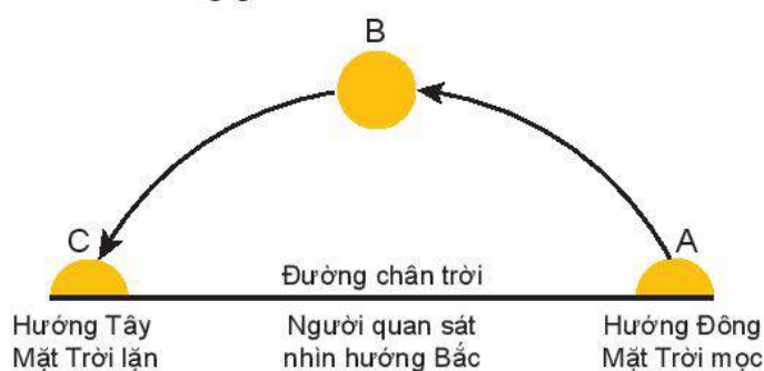
Hình 5.3. Hình ảnh nhìn thấy đường đi của Mặt Trời quan sát từ Trái Đất
