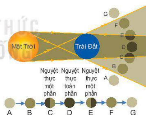
Hình 6.9. Các pha nguyệt thực
