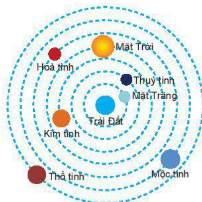
Hình 5.13. Mô hình hệ địa tâm của Ptolemy
