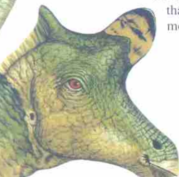
Lambeosaurus
