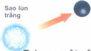
Sao lùn đen chết
