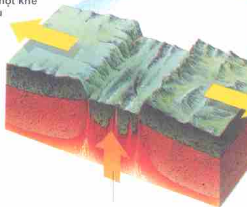
Đá nóng chảy dâng lên để lấp đầy khe nứt ở đáy đại dương
