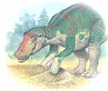
Một số trứng khủng long có vỏ sần sùi trong khi số khác lại nhẵn nhụi
