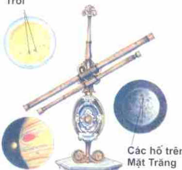
Sao Mộc
