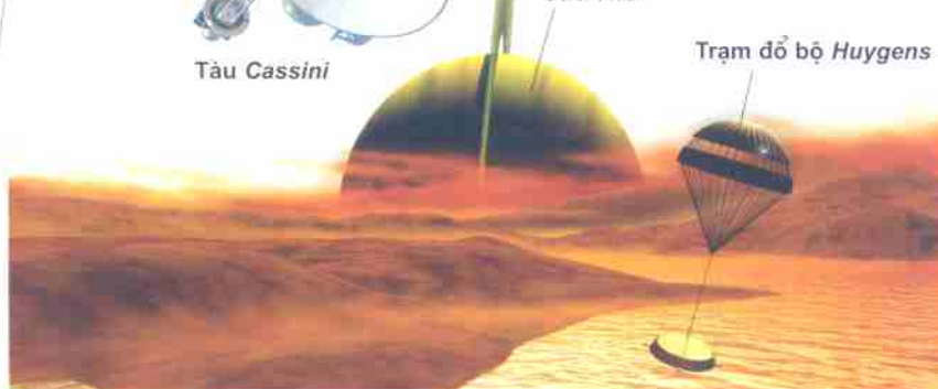
Sao Thổ
