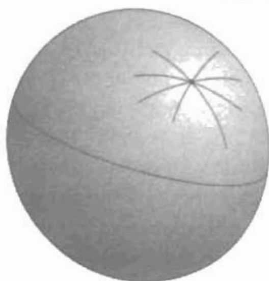
Hình 28: Tập hợp các vòng tròn lớn qua một điểm.
