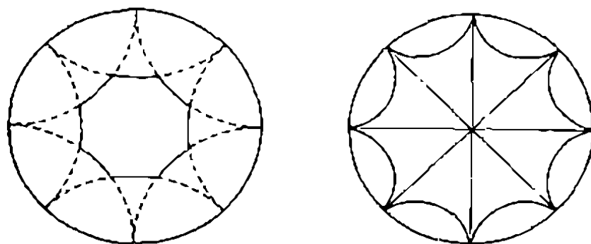
Hình 47 Bát giác ở bên trái có các góc lớn hơn 90 độ. Bát giác ở bên phải có các góc bằng 0 độ. Nếu bát giác ở bên trái từ từ to ra các góc của nó sẽ thu nhỏ lại dần, ta sẽ có được một bát giác với các góc bằng 45 độ trước khi nó biến thành bát giác bên phải.
