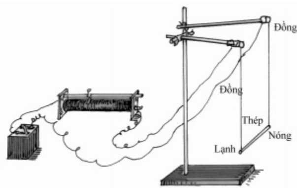
Hiệu ứng Peltier
