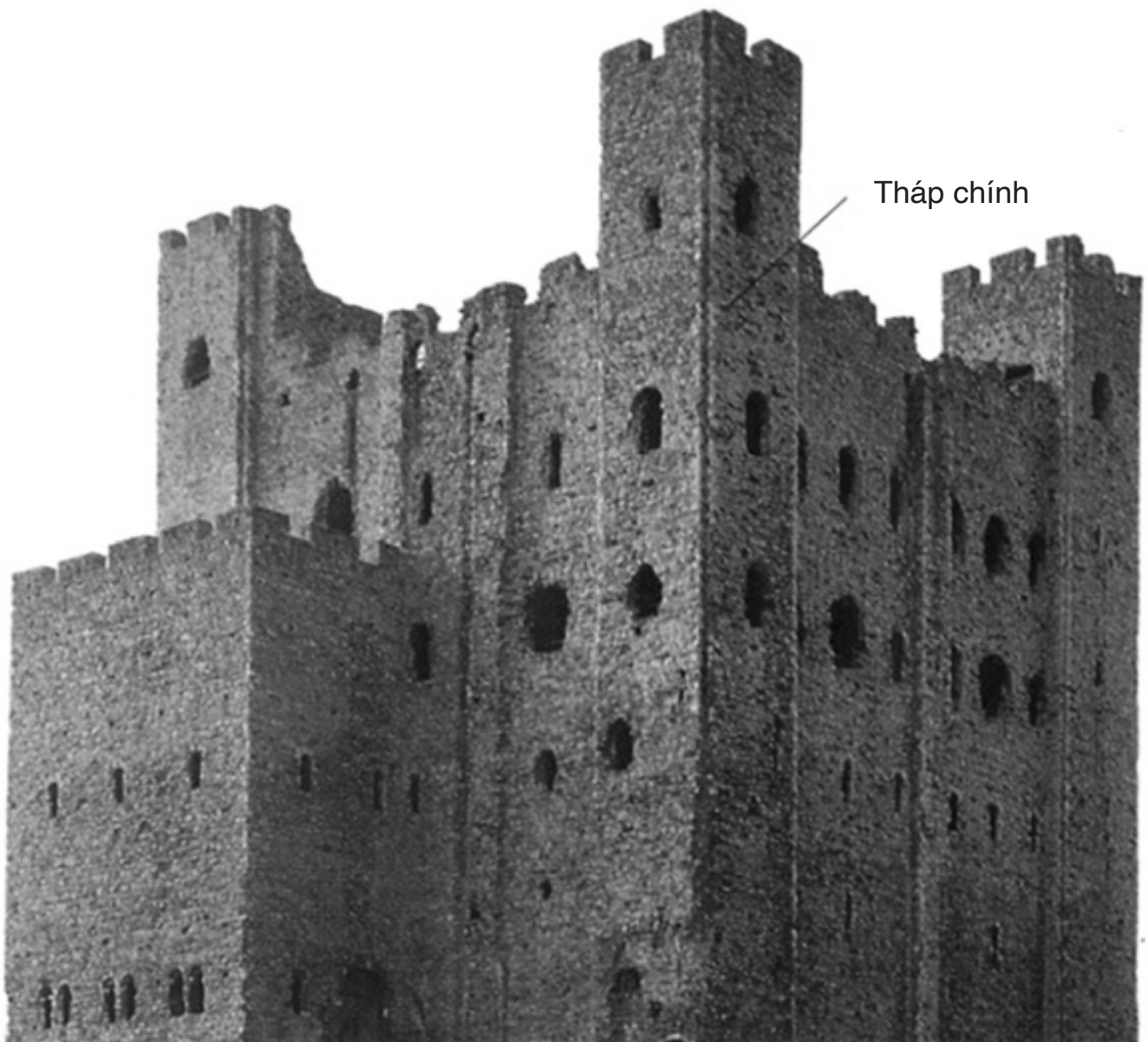
Lâu đài Rochester ở Anh
