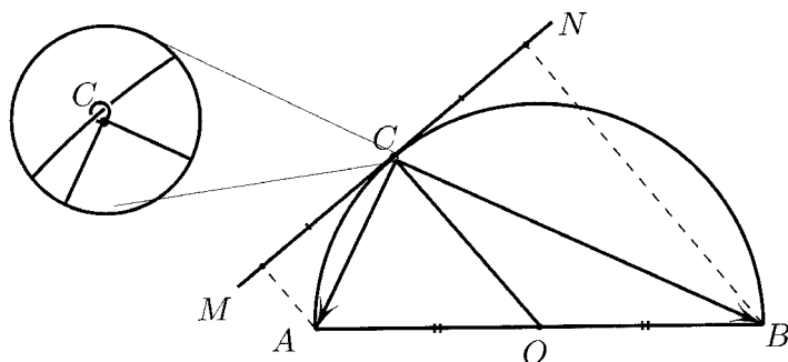
Hình 2.11. Chứng minh cho bởi những lò xo.
