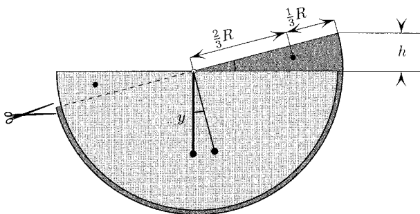
Hình 5.2. Độ nặng của tâm khối hình quạt là 2/3h , trong đó h là độ nặng của cung.
