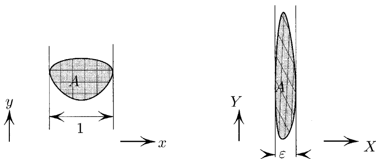
Hình 9.4. Nén phạm vi của x làm giãn phạm vi của y , dẫn theo điều kiện bảo toàn diện tích.
