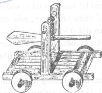
Hình 53. Gỗ húc ở trên xe húc
