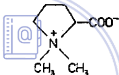
Stachydrin
