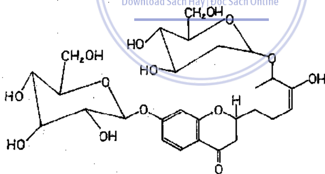
Butrin
