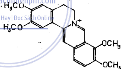
Palmatin
