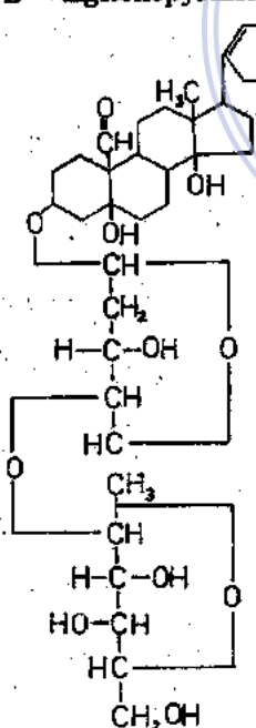
Olitorisid
