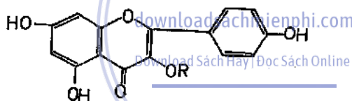
Kaempferol
