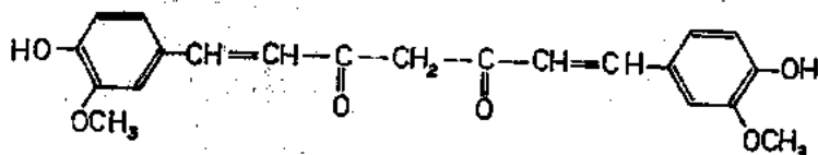
Curcumin
