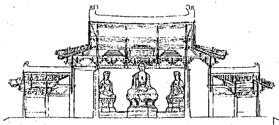
272. Mặt cắt dọc điện Moni chùa Long Heng
