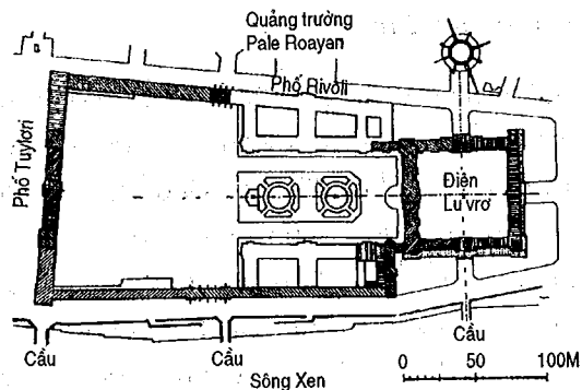
244. Điện Luvơ - Mặt nhà và vị trí bên sông Xen
