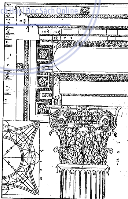
119. Thức cột phức hợp (Composít)
