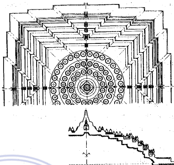
306. Mặt bằng, mặt cắt đền Bôrôbudua
