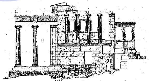
89. Đền Eréchtayôn - Mặt bằng, mặt nhà và mặt cắt
