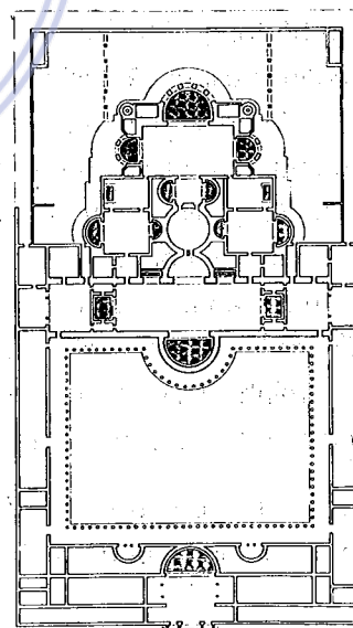
Terma Hoàng gia ở Rôma Mặt bằng vị trí (trên) và mặt bằng công trình (bên)
