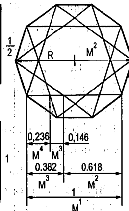
387. Xây dựng tỷ lệ trong kiến trúc cổ và cách dùng tỷ lệ vàng
