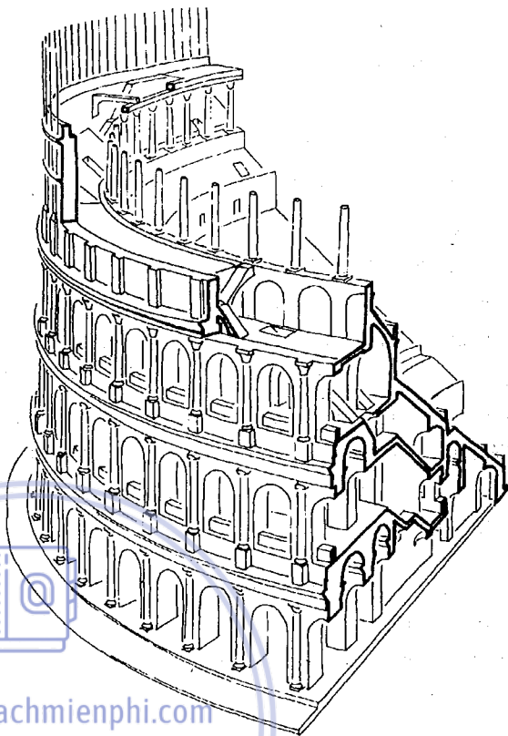
140. Cấu trúc đấu trường Côlôđê
