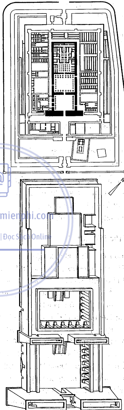
54. Tổng mặt bằng và phối cảnh đền thờ Ramxes III ở Ambuximbel 1175 trước Công nguyên
