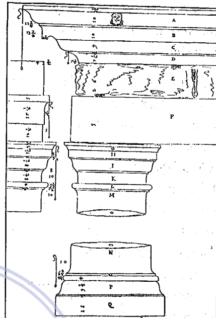
118. Thức cột Toscan - La Mã
