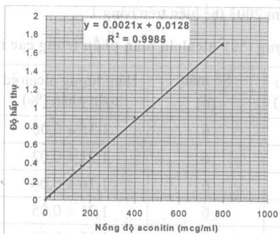
Hình 3. Đường cong chuẩn định lượng diester alcaloid tính theo aconitin
