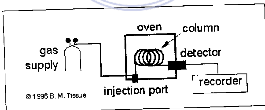
Hình 14: Sơ đồ cấu tạo máy SKK
