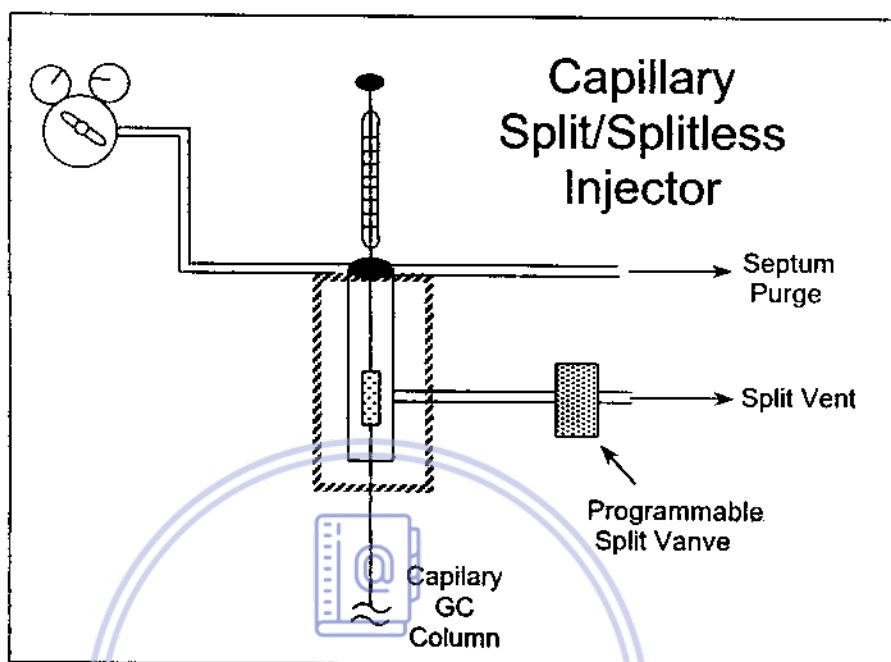
Hình 16: Sơ đồ cổng bơm chia và không chia dòng
