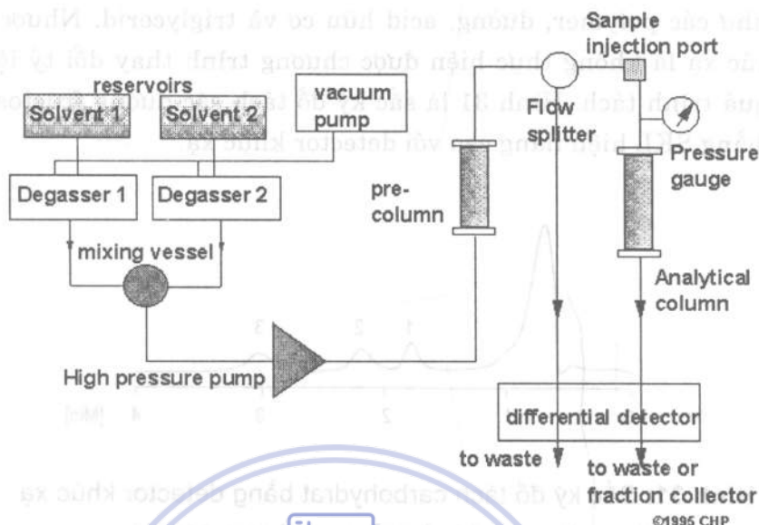
Hình 30: Sơ đồ cấu tạo SKL hiệu năng cao
