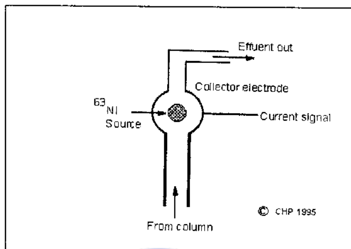
Hình 21: Sơ đồ cấu tạo detector cộng kết điện tử
