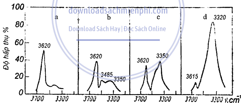
Hình 13: Những phổ hồng ngoại của hợp chất chứa hydroxyl:
