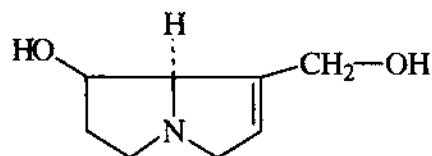
Retronecin
