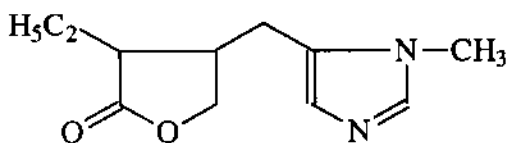
Pilocarpin
