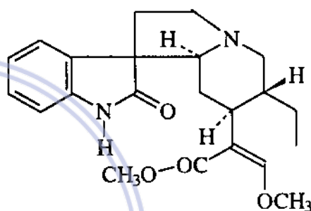
Rhyncophyllin
