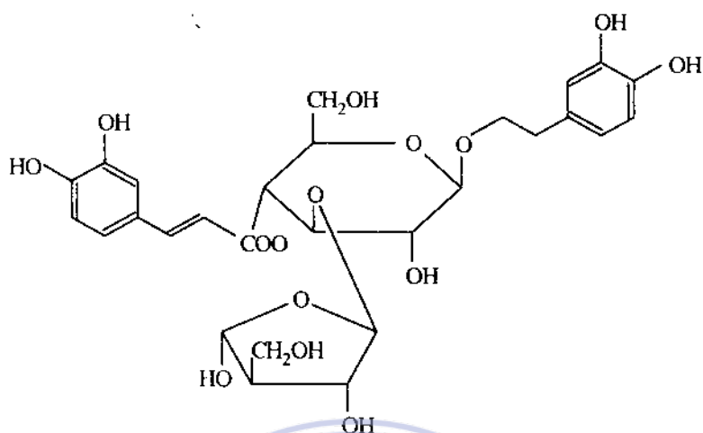
Nuomiosid A
