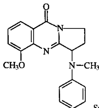
Isofebrifugin
