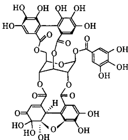
Geraniin
