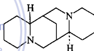
Sparteïn
