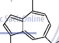
Chamazulen
