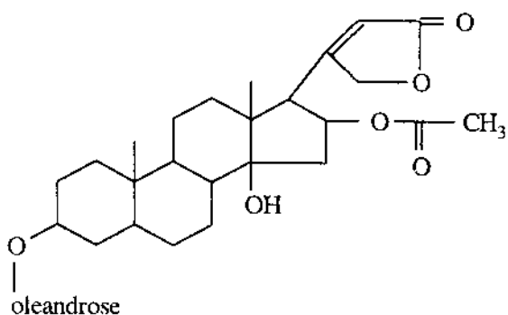
Oleandrin
