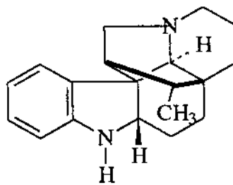
Tuboxenin
