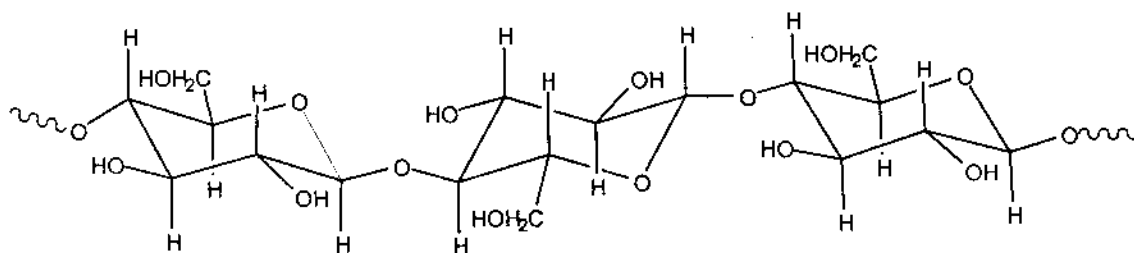
Cellulose
