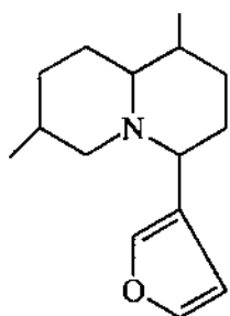
Desoxynupharidin
