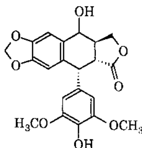
\alpha -Pelatin
