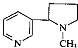
Nicotin
