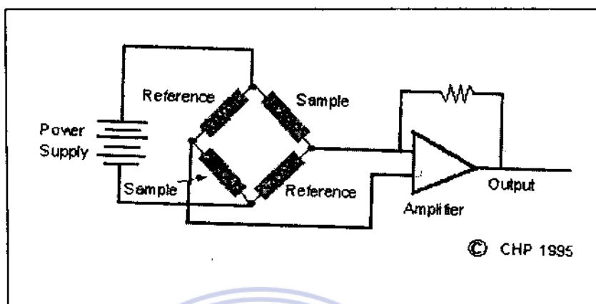
Hình 20: Sơ đồ cấu tạo detector dẫn nhiệt
