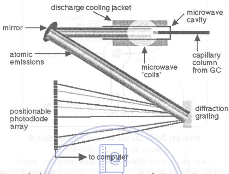
Hình 22: Sơ đồ cấu tạo detector phát xạ nguyên tử [Thomas G. Chasteen, Sam Houston State University, Huntsville, Texas 77341, 17/9/2003:
