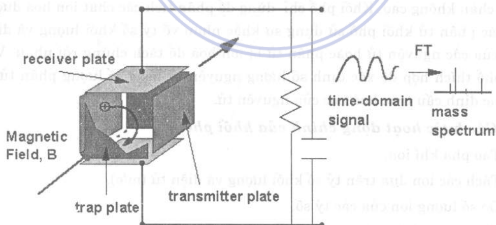
Hình 26: Sơ đồ cấu tạo bộ phận phân tích khối phổ chuyển khối
