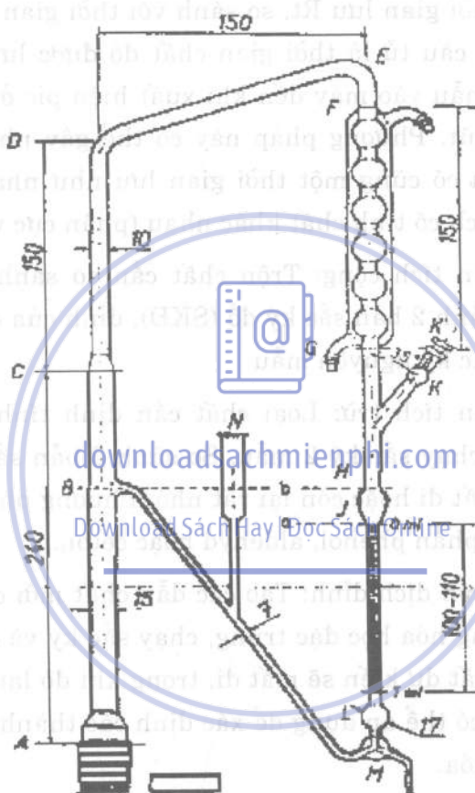
Dụng cụ định lượng tinh dầu trong dược liệu theo Dược điển Viện Nam III (đơn vị đo: mm)
