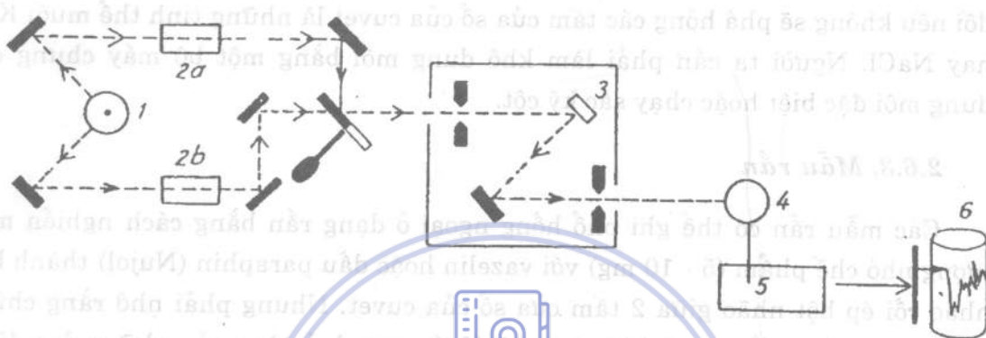
Hình 18: Sơ đồ chung của phổ kế hồng ngoại:
