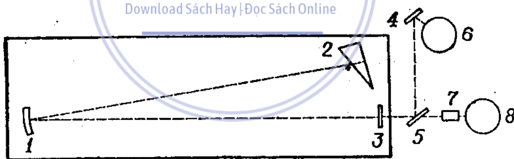
Hình 1. Sơ đồ quang học của máy quang phổ Beckman DU cấu tạo theo nguyên lý một chùm tia:
