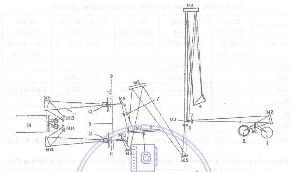
Hình 2. Sơ đồ quang học của máy quang phổ Unicam SP-800
