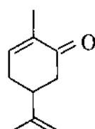
Carvon
