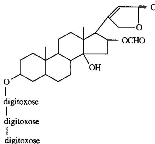
Gitaloxin
