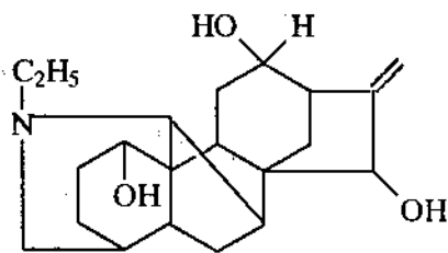
Napellin
