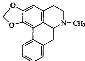
Roemerin
