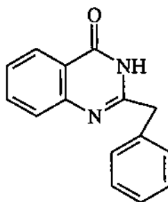
Glycosminin
