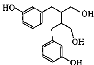
Enterodiol
