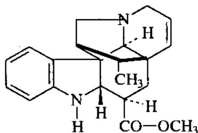
Vindolinin
