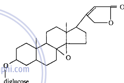
Adynerin
