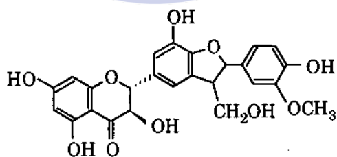
Silychristin
