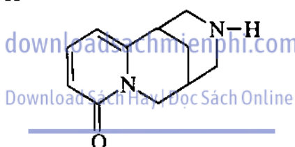
Cytisin
