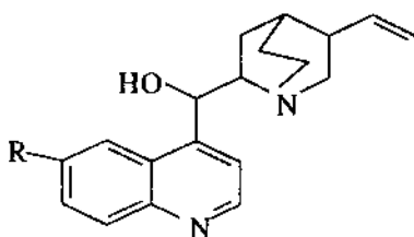
Kiểu Cinchonin
