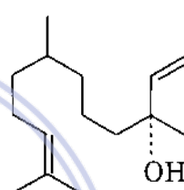
Nerolidol
