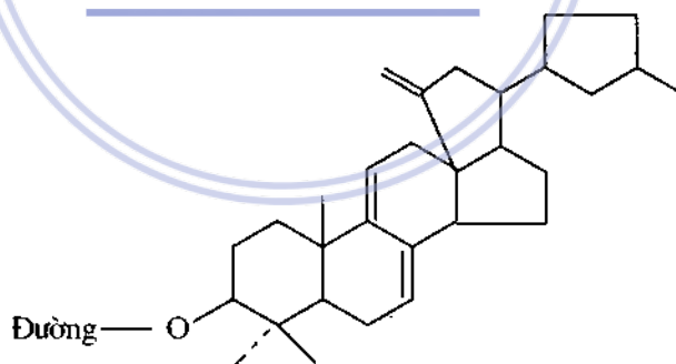
Holothurin A
