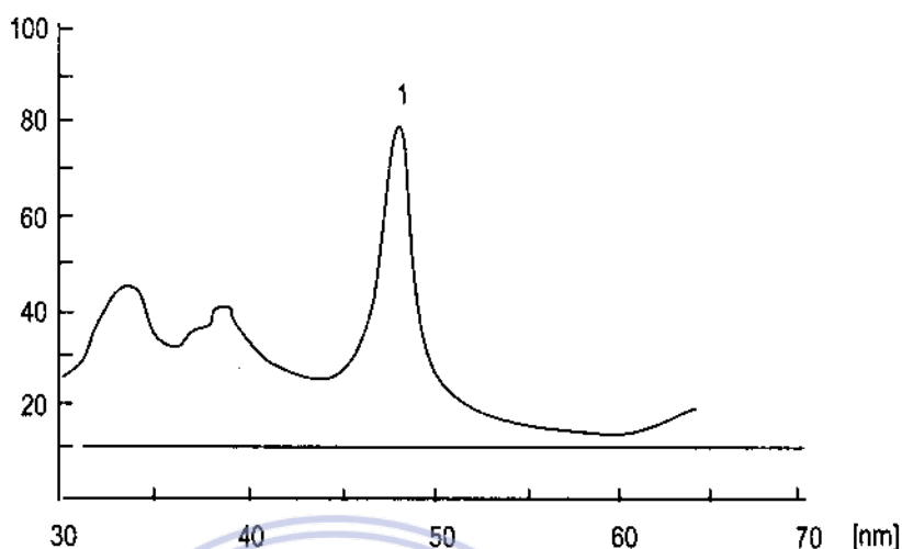
Hình 6 : Phổ densitomet của thujon từ Salvia fruticosa (do Viện nghiên cứu Thuốc thú y - Berlin - Đức nghiên cứu và công bố năm 1996)
