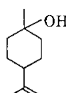
Terpineol
