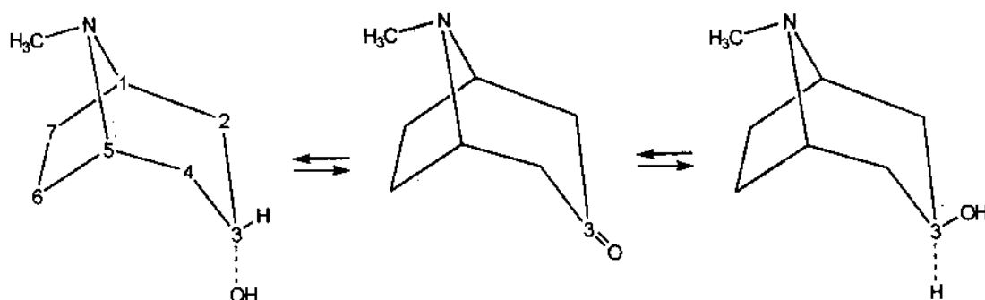
Tropin (F : 63°)
