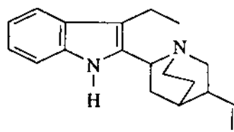
Kiểu Cinchonamin
