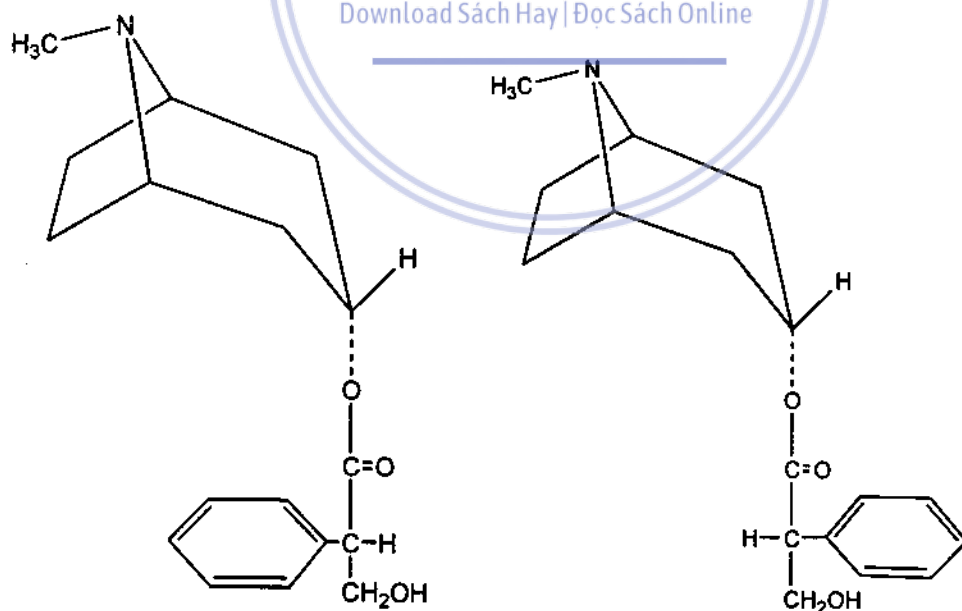
l - Hyoscyamin
