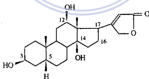
Digoxigenin
