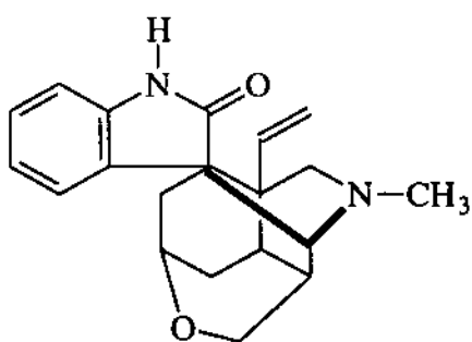
Gelsemin
