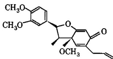
Kadsurenol
