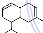
cadinen
