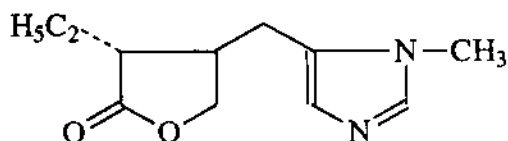
Isopilocarpin
