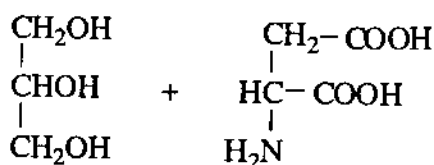
Glycerin
