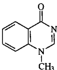
Glycorin
