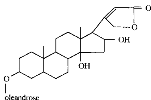
Desacetyl oleandrin
