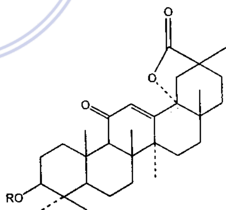
Isoglabrolid
