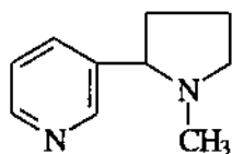
Nicotin
