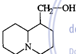
Lupinin
