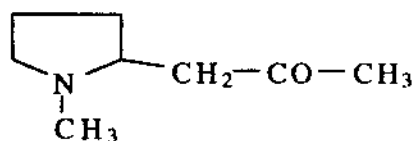
Hygrin
