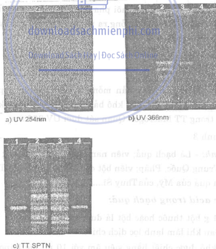
Hình 3: SKLM hiệu năng cao lá bạch quả ( Ginkgo biloba )
