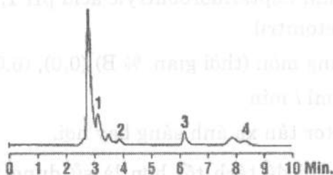
Hình 43: Tách các acid hữu cơ [www.alltechweb.com.chromcccess]:
