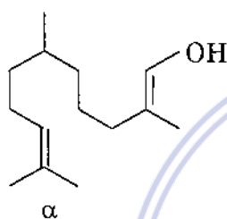
Farnesol
