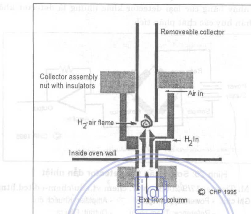
Hình 19: Sơ đồ detector ion hoá ngọn lửa
