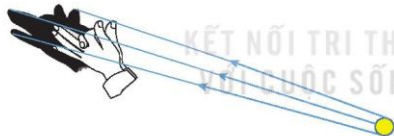
Hình 15.2a. Bóng đen gây bởi bóng đèn tròn (nguồn sáng hẹp)
