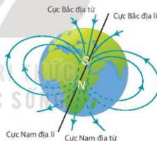
Hình 19.7 Mô phỏng từ trường Trái Đất
