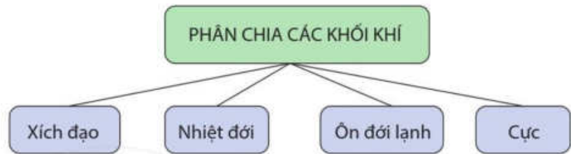
Hình 13.3. Các khối khí chính
