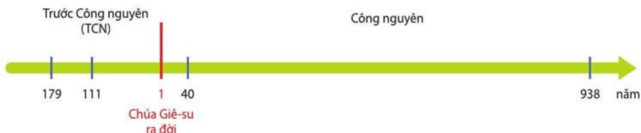
Hình 2.3. Sơ đồ thời gian theo Công lịch
