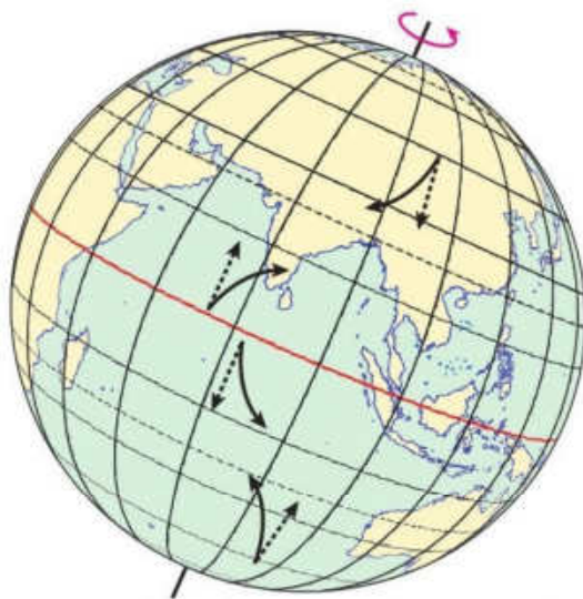
Hình 6.5. Sự lệch hướng chuyển động của các vật thể ở bán cầu Bắc và bán cầu Nam
