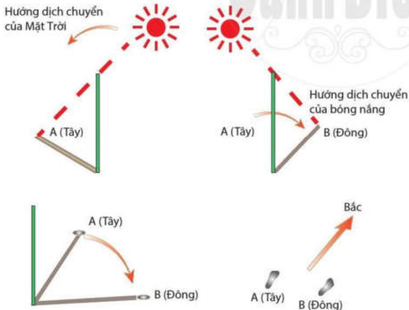
Hình 8.3. Xác định phương hướng khi quan sát sự dịch chuyển của bóng nắng
