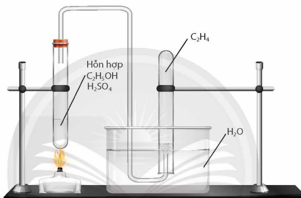
▲ Điều chế và thu khí ethylene trong phòng thí nghiệm
