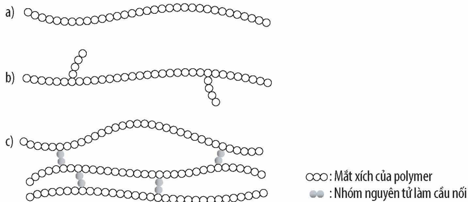
▲ Mô hình cấu tạo polymer
