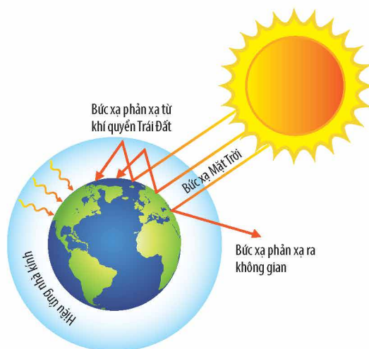
▲ Hiệu ứng nhà kính
