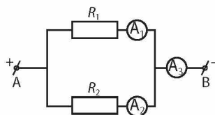
▲ Sơ đồ một đoạn mạch điện gồm hai điện trở mắc song song
