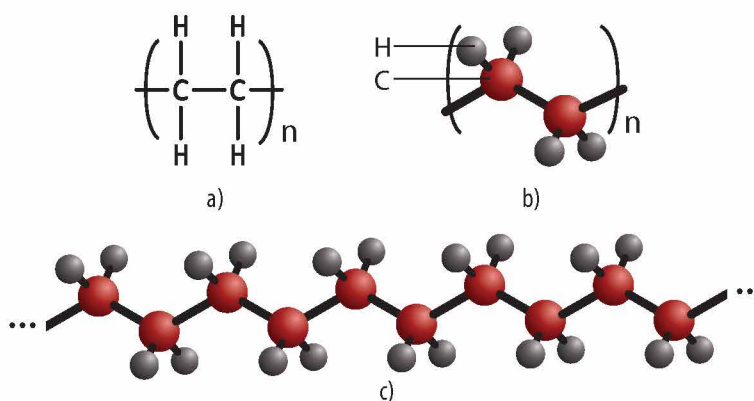
▲ a) Công thức cấu tạo ethylene; b) Mô hình cấu tạo ethylene; c) Mô hình cấu tạo khai triển ethylene
