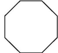
Bát giác đều
