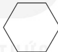
Lục giác đều
