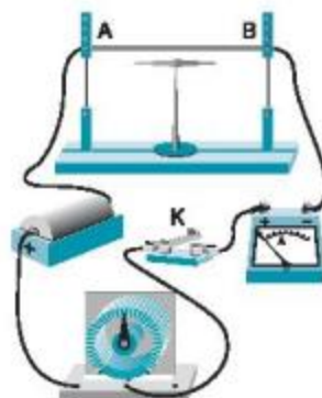
Hình 19.1 Thí nghiệm Osterd
