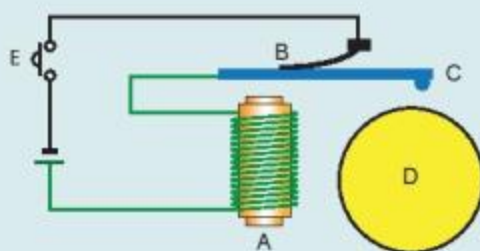
Hình 20.4 Sơ đồ cấu tạo chuông điện
