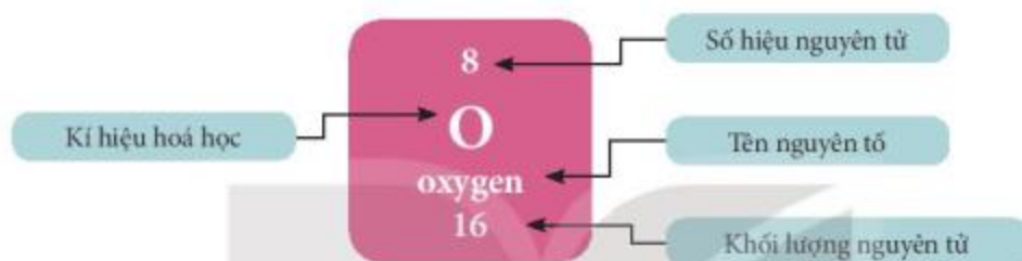
Hình 4.2 Ô nguyên tố oxygen
