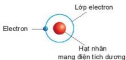
a) Nguyên tử hydrogen
