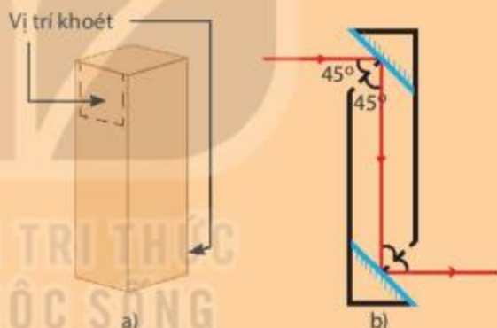
Hình 16.7 Dụng cụ làm kính tiềm vọng
