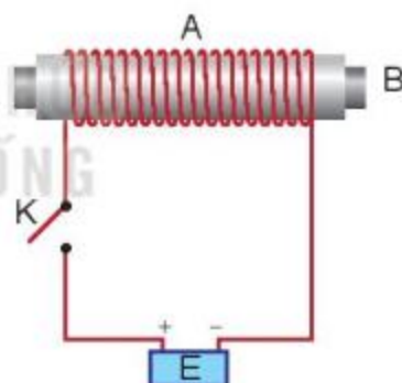
Hình 20.1 Cấu tạo của nam châm điện
