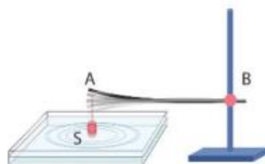
Hình 12.2 Sóng truyền trên mặt nước
