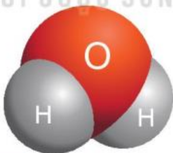
Hình 29.1 Mô hình cấu tạo phân tử nước
