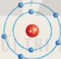
Hình 4.4 Mô hình sắp xếp các electron ở vỏ nguyên tử nitrogen
