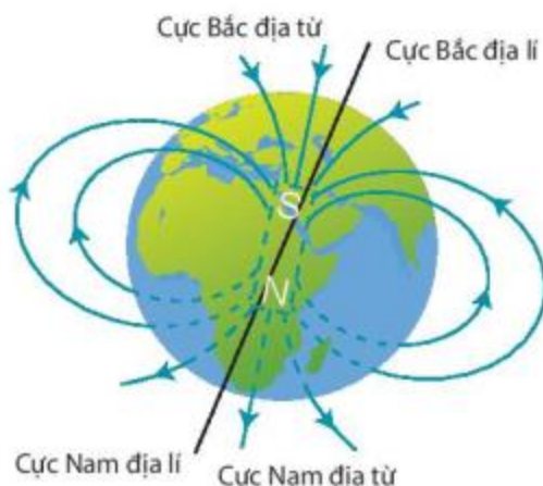
Hình 19.7 Mô phỏng từ trường Trái Đất
