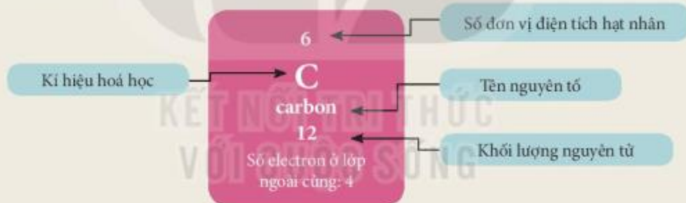
Hình 4.1 Các thông tin về nguyên tố carbon
