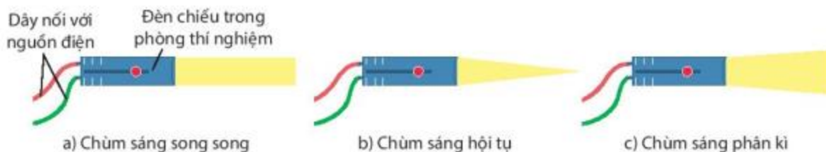
Hình 15.3 Các loại chùm sáng
