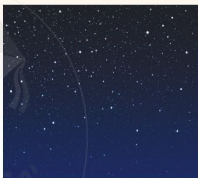
Hình 35.1. Bầu trời đêm
