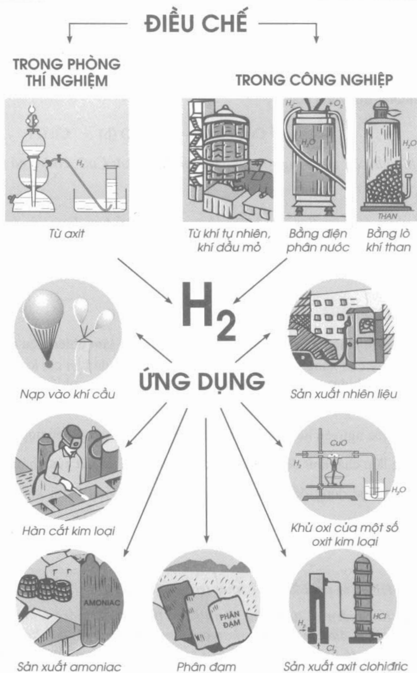
Hình 5.3 Điều chế và ứng dụng của hidro
