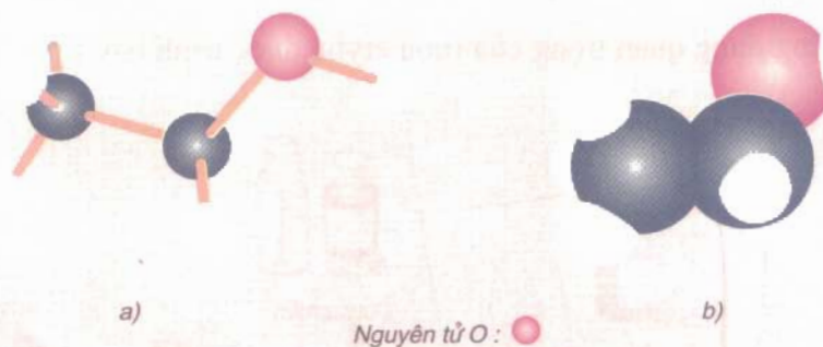
Hình 5.2. Mô hình phân tử rượu etylic: a) Dạng rắn ; b) Dạng lỏng
