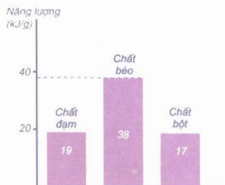
Hình 5.8. So sánh năng lượng toả ra khi oxi hoá thực ăn
