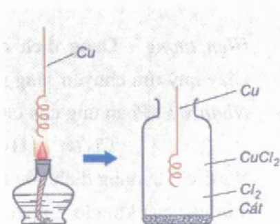
Hình 3.2. Đồng tác dụng với clơ
