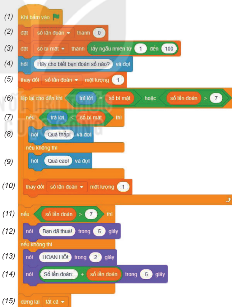
Hình 15.4. Chương trình cần được gỡ lỗi
