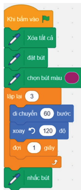
Hình 12.4. Chương trình vẽ hình tam giác đều
