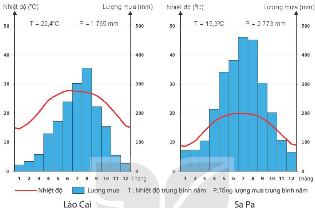
Hình 4.2. Biểu đồ nhiệt độ, lượng mưa tại trạm khí tượng Lào Cai (độ cao 104 m) và trạm khí tượng Sa Pa (độ cao 1 583 m) thuộc tỉnh Lào Cai
