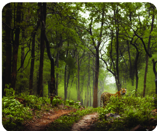
Hình 2. Mùa mưa ở rừng nhiệt đới gió mùa Ben-gan
