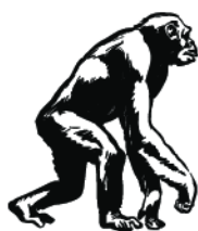
Vượn người
