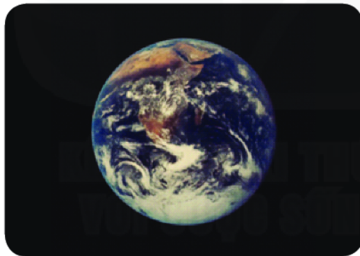
Hình 2. Một số bằng chứng về dạng khối cầu của Trái Đất
