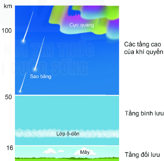
Hình 1. Các tầng khí quyển
