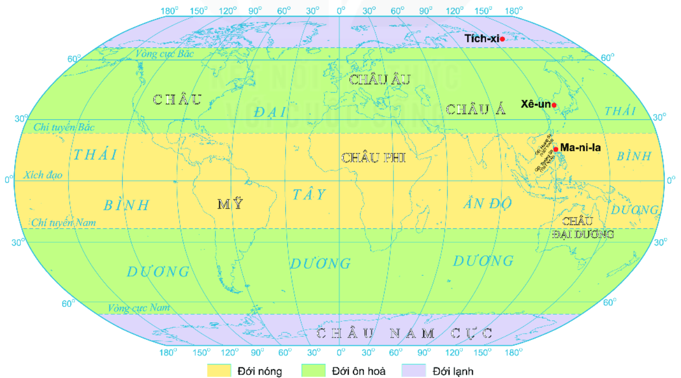
Hình 2. Các đới khí hậu trên Trái Đất
