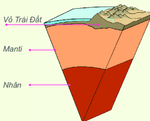
Hình 1. Lát cắt về cấu tạo Trái Đất
