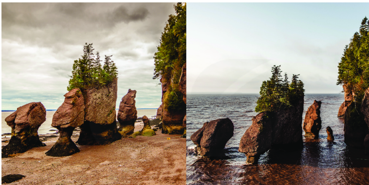
Hình 2. Hiện tượng thủy triều ở vịnh Phăng-đi (Ca-na-đa)
