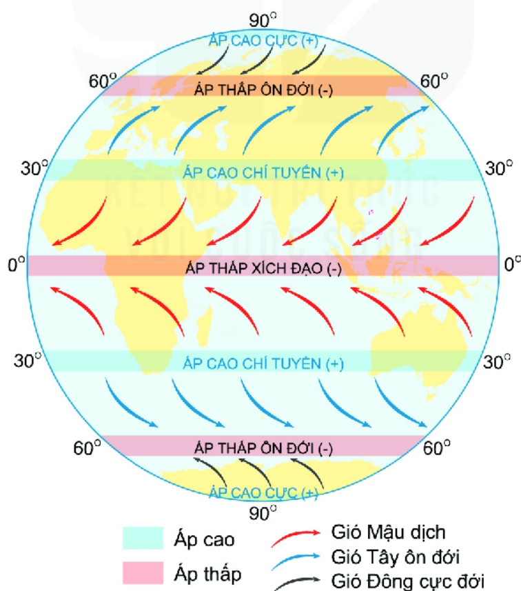
Hình 5. Các đai khí áp và gió chính trên Trái Đất
