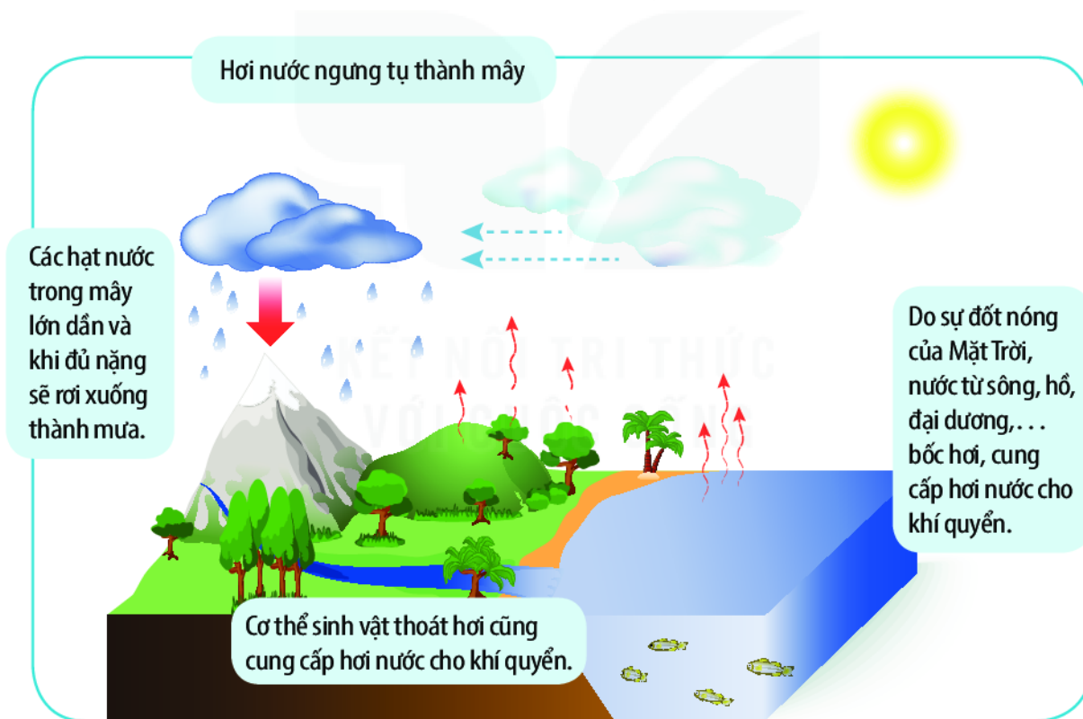
Hình 5. Quá trình hình thành mây và mưa
