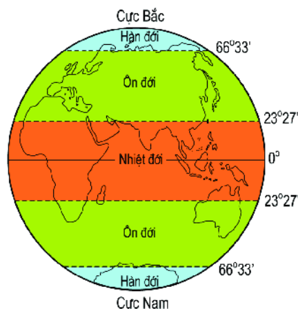
Hình 1. Các đới khí hậu trên Trái Đất
