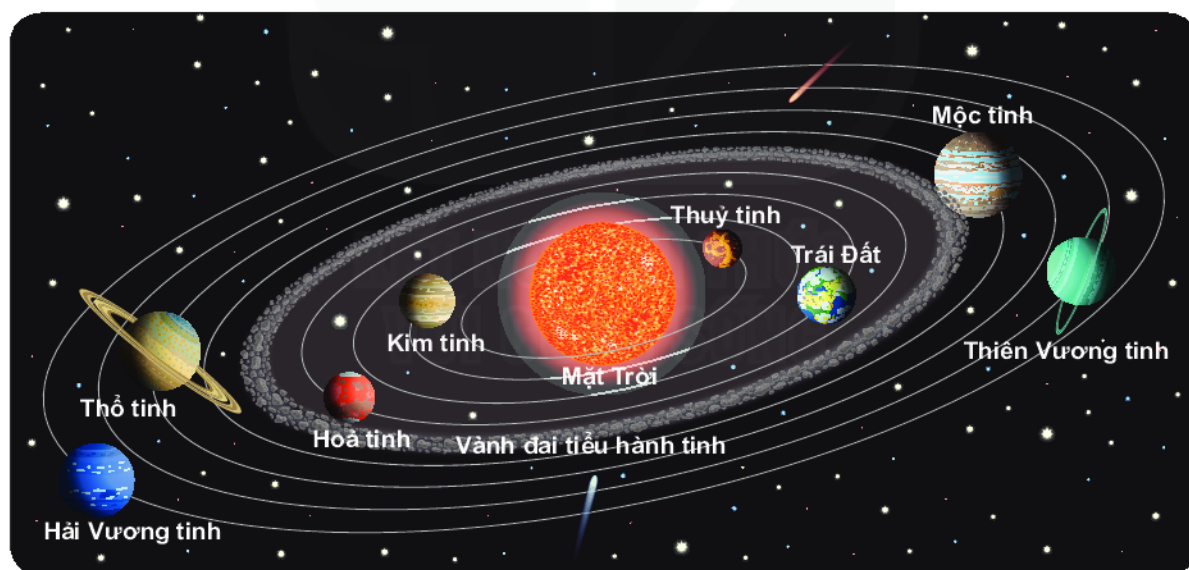
Hình 1. Các hành tinh trong hệ Mặt Trời
