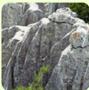
Đá vôi
