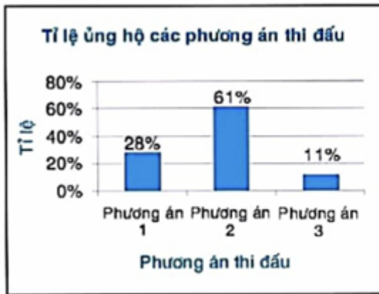
Hình 1. Biểu đồ cột
