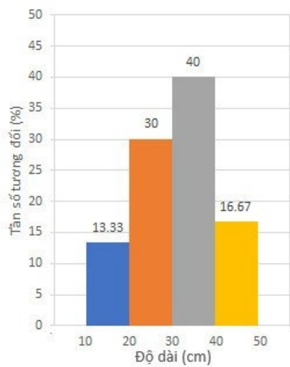
Biểu đồ tần số tương đối ghép nhóm ở dạng biểu đồ cột
