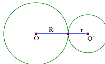
Hình 2: Tiếp xúc ngoài.
