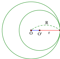
Hình 1: Tiếp xúc trong.
