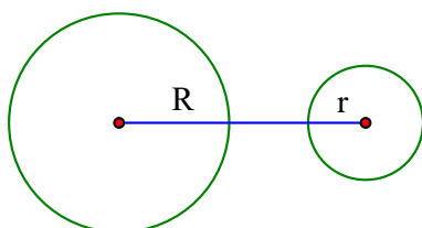
Hình 1: Hai đường tròn ngoài nhau.
