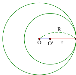
Hình 1: Tiếp xúc trong.
