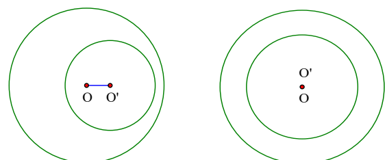
Hình 2: Hai đường tròn đựng nhau.
