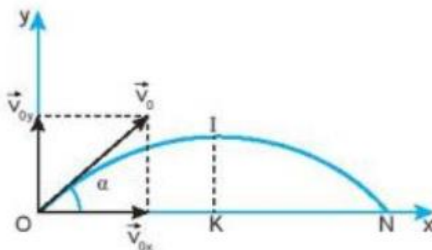
Hình 12.5. Phân tích chuyển động ném xiên
