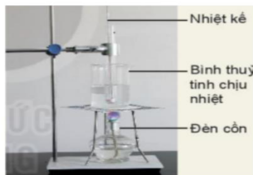
Hình 2.2: Thí nghiệm đo nhiệt độ sôi của nước
