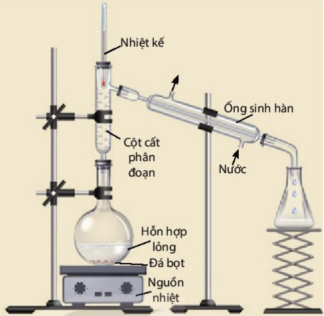
Hình 11.3. Thiết bị, dụng cụ tách chất bằng phương pháp chưng cất phân đoạn
