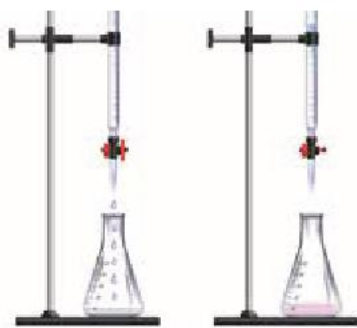
Hình 2.6. Chuẩn độ dung dịch NaOH bằng dung dịch HCl Hình 2.7. Thao tác khi chuẩn độ
