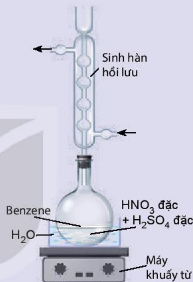
Hình 17.2. Thí nghiệm nitro hoá benzene
