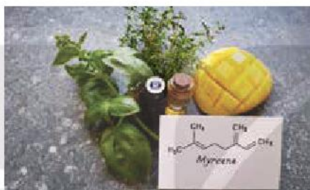
c) Myrcene (có trong lá húng quế, cỏ xạ hương, quả xoài)
