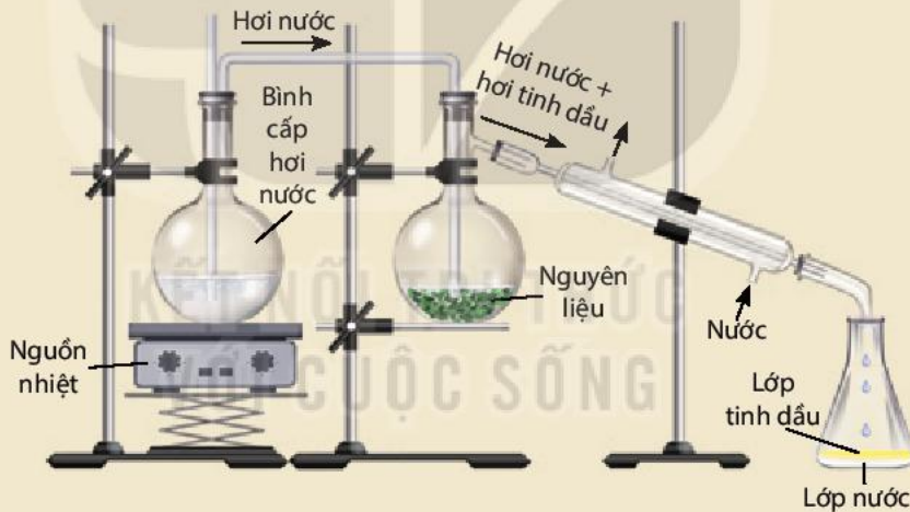
Hình 11.4. Thiết bị, dụng cụ chưng cất lôi cuốn hơi nước
