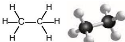
b) ethane
