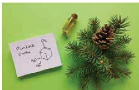
a) Pinene (có trong nhựa thông)
