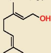
geraniol (tinh dầu hoa hồng)
