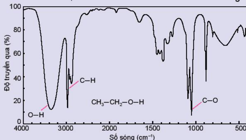
Hình 10.2. Phổ hồng ngoại của ethanol
