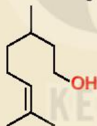
citronellol (tinh dầu sả)
