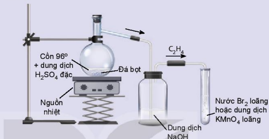
Hình 16.5. Điều chế ethylene và thử tính chất
