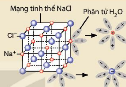
Hình 2.3. Mô hình biểu diễn sự phân li của NaCl trong nước
