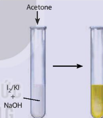
Hình 23.7. Phản ứng iodoform
