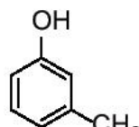
m-cresol
