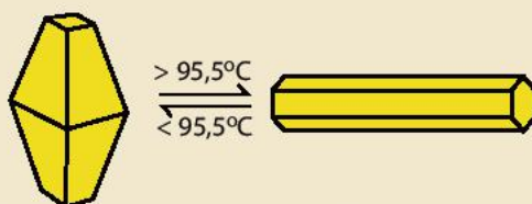
Hình 7.4. Tinh thể sulfur
