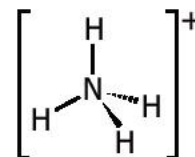
Hình 5.3. Dạng hình học của ion ammonium
