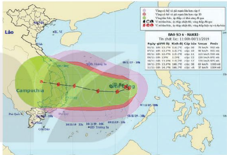
Hình 4.31. Ta có thể dùng một phần mặt phẳng toạ độ để mô tả một phạm vi nhất định trên Trái Đất mà vị trí x^\circ vĩ bắc, y^\circ kinh đông của tâm áp thấp được thể hiện bởi điểm có toạ độ (x; y) .
