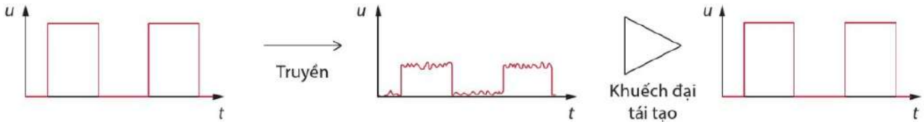
Hình 2.3. Tín hiệu số bị nhiễu và suy giảm trong quá trình truyền; được khôi phục khi khuếch đại tái tạo
