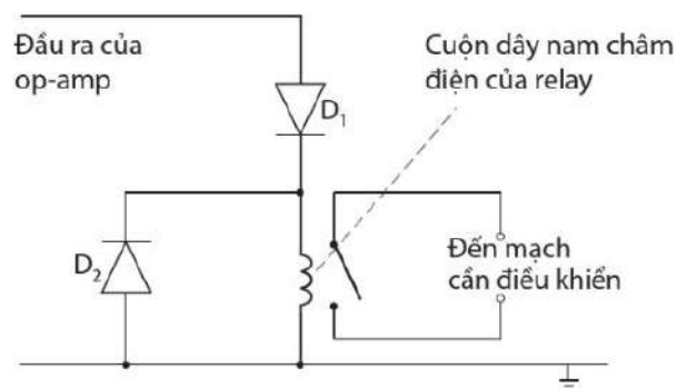
Hình 2.7. Sơ đồ nguyên lý mạch op-amp – relay
