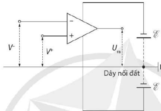
Hình 1.14. Sơ đồ nguyên tắc dùng op-amp như bộ so sánh điện thế
