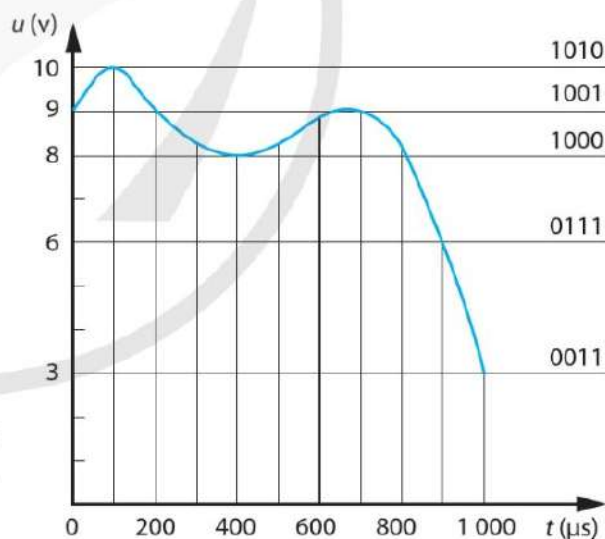
Hình 2.5. Quá trình lấy mẫu (Đường màu xanh biểu diễn sự thay đổi hiệu điện thế u theo thời gian t và là tín hiệu tương tự)
