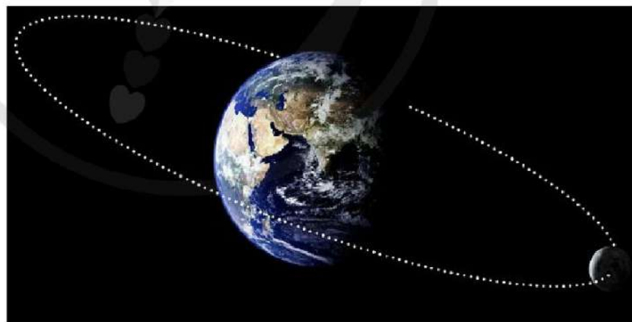
Hình 1.5. Mặt Trăng chuyển động trong trường hấp dẫn của Trái Đất (hình vẽ không theo đúng tỉ lệ)
