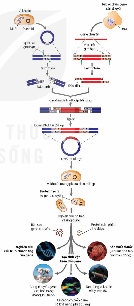
Hình 5.1. Tóm tắt nguyên lí tạo DNA tái tổ hợp ở vi khuẩn E. coli và ứng dụng thực tiễn
