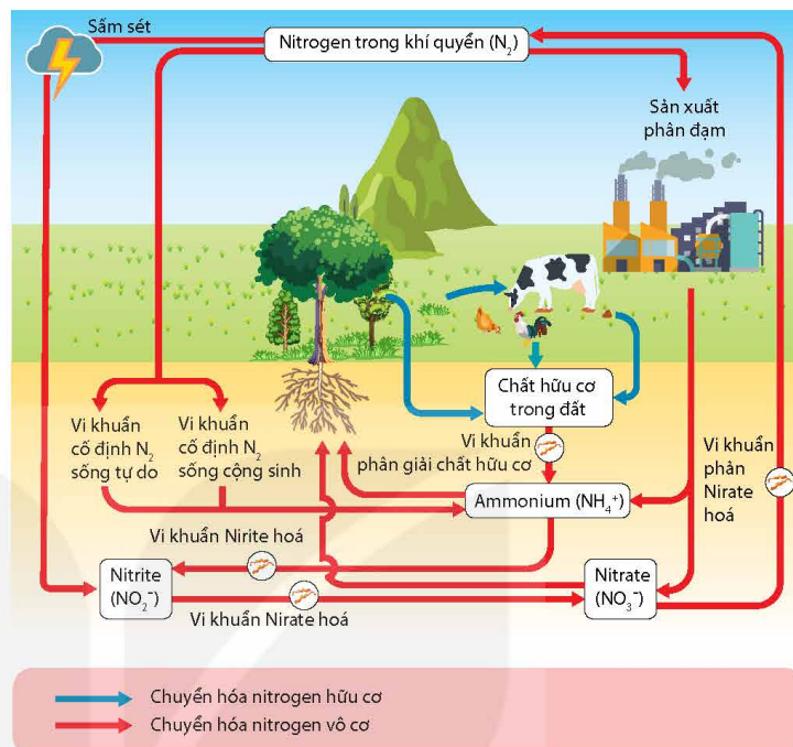
Hình 31.6. Chu trình nitrogen
