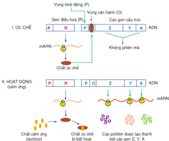
Hình 3. Sơ đồ cơ chế điều hoà hoạt động của operon Lac ở E. coli
