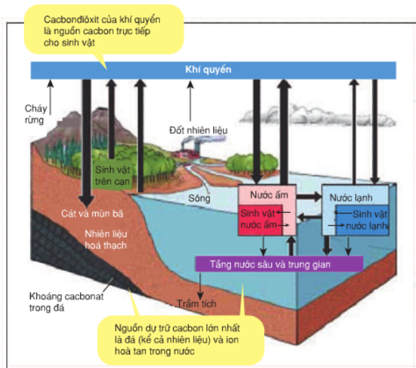
Hình 61.3. Chu trình cacbon toàn cầu
