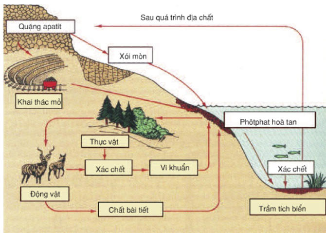
Hình 61.6. Chu trình photpho trong tự nhiên
