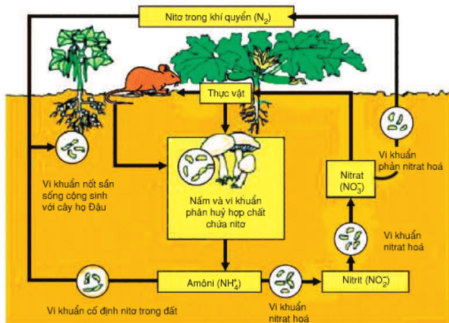
Hình 61.4. Sơ đồ chu trình nitơ
