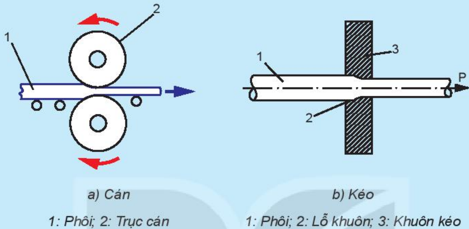
Hình 3.5. Sơ đồ cán, kéo kim loại
