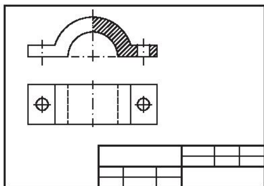
Hình 14.5. Vẽ mờ
