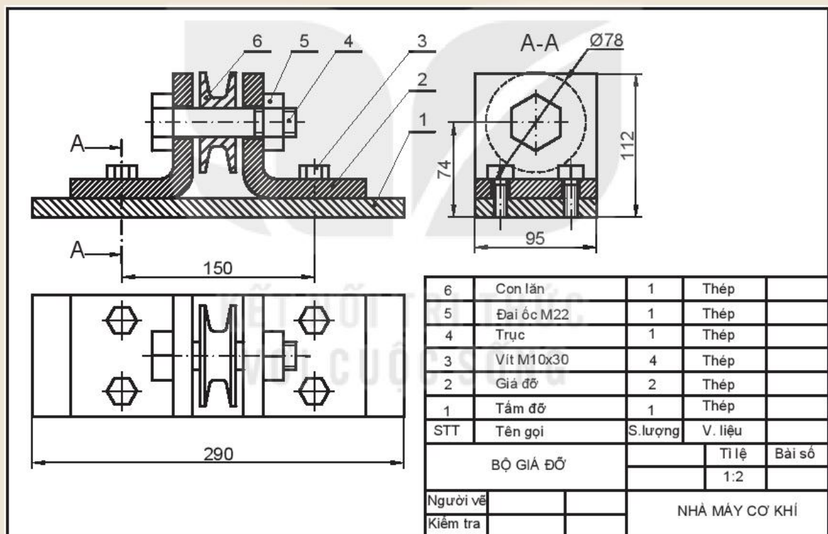
Hình 14.8. Bản vẽ lắp bộ giá đỡ
