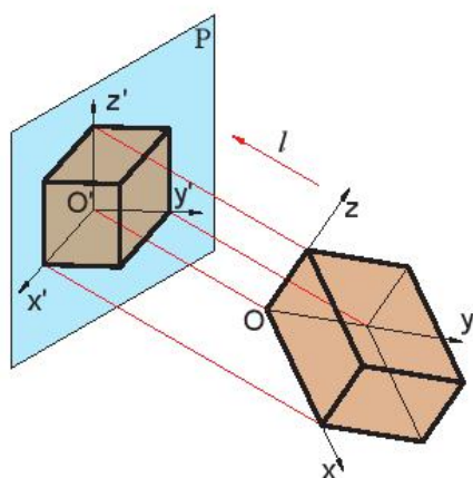
Hình 11.4. Hình chiếu trực đo vuông góc đều
