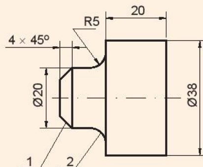
Hình 16.4. Trục
