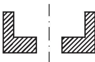
Hình 10.15. Mặt cắt
