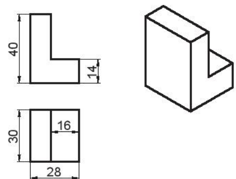
Hình 12.5. Giá chữ L
