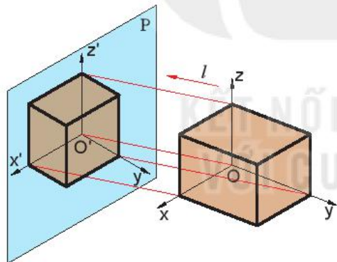
Hình 11.9. Hình chiếu trục đo xiên góc cân
