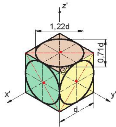
Hình 11.6. Các elip trong HCTĐ vuông góc đều
