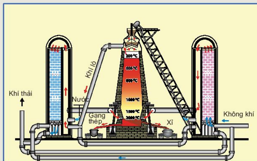
Hình 3.2. Sản xuất gang – thép trong lò cao
