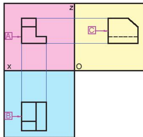
Hình 9.5. Các hình chiếu vuông góc
