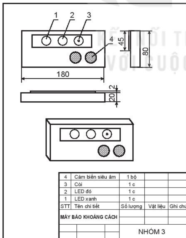
a) Bản vẽ lắp
