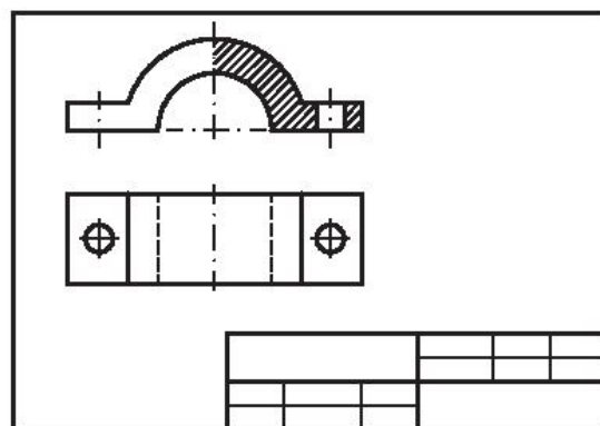
Hình 14.6. Tô đậm
