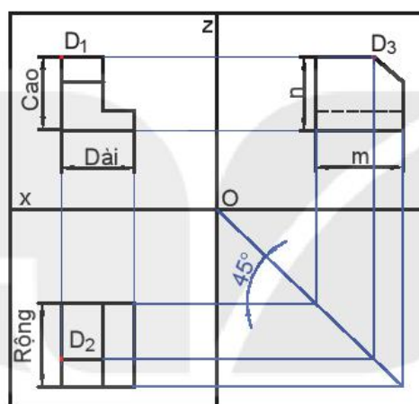
Hình 9.6. Mối quan hệ giữa ba hình chiếu
