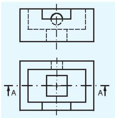
Hình 10.10. Giá đỡ
