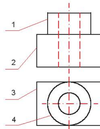
Hình 16.3. Gối đỡ
