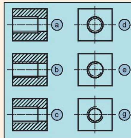
Hình 13.9. Ren lỗ
