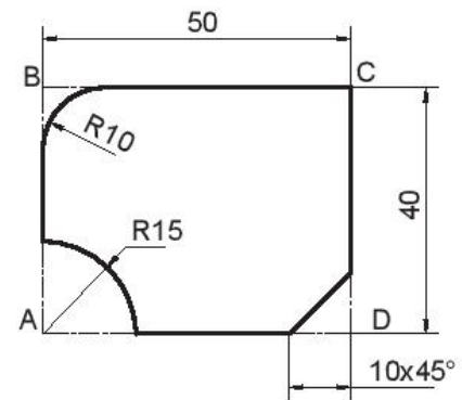
Hình 16.5. Tấm phẳng
