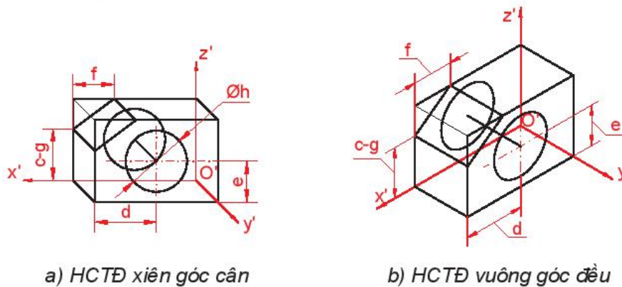
Hình 11.16. Vẽ các thành phần của vật thể
