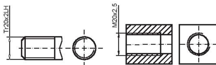
Hình 13.10. Ghi kích thước ren
