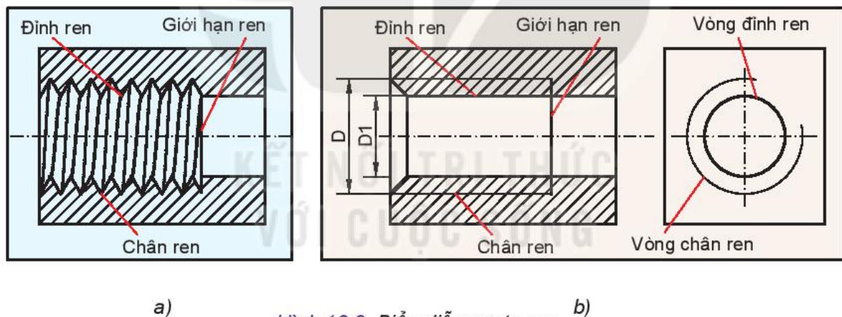
Hình 13.6. Biểu diễn ren trong
