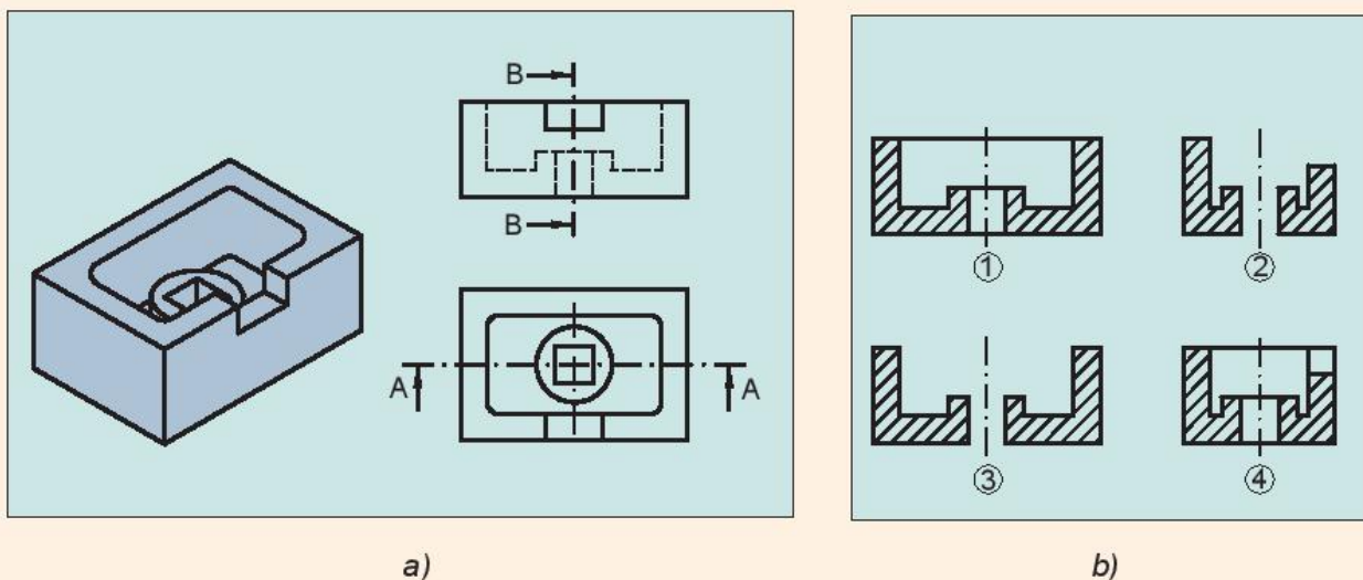
Hình 10.5. Thân máy: a) Các hình chiếu; b) Hình cắt, mặt cắt
