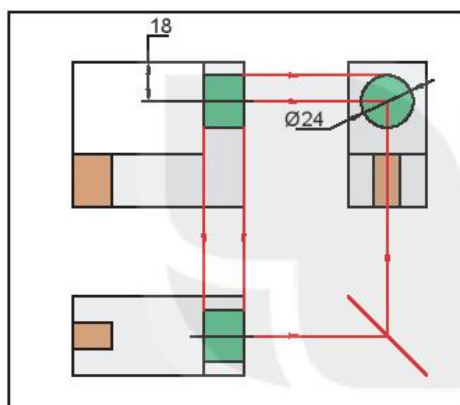
Hình 9.15. Vẽ lỗ trụ
