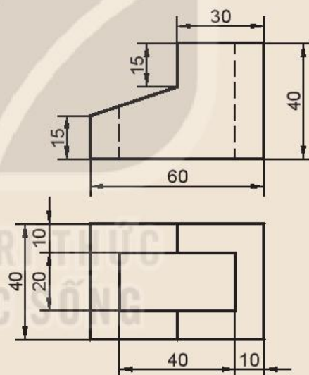
Hình 11.19. Đế
