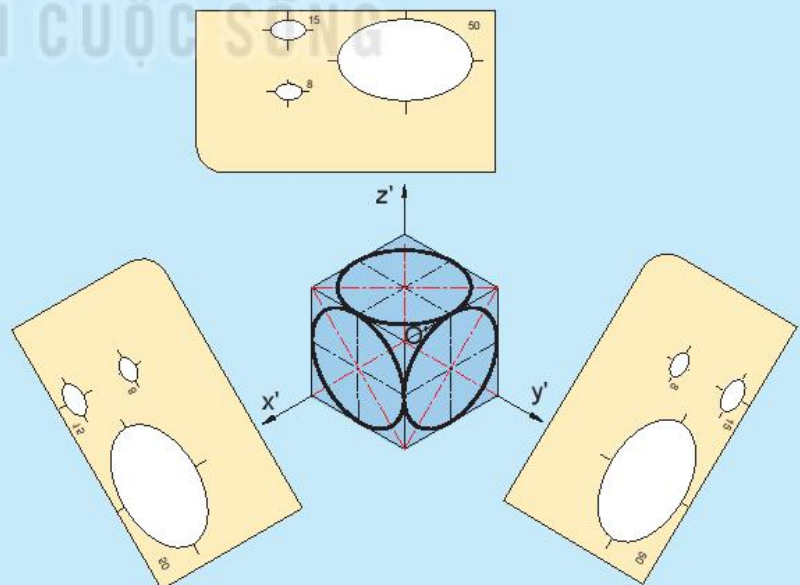
Hình 11.7. Cách đặt thước elip để tô
