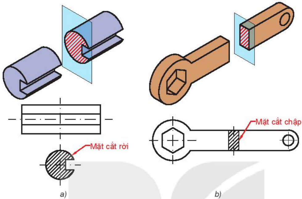
Hình 10.9. Mặt cắt rời và mặt cắt chập
