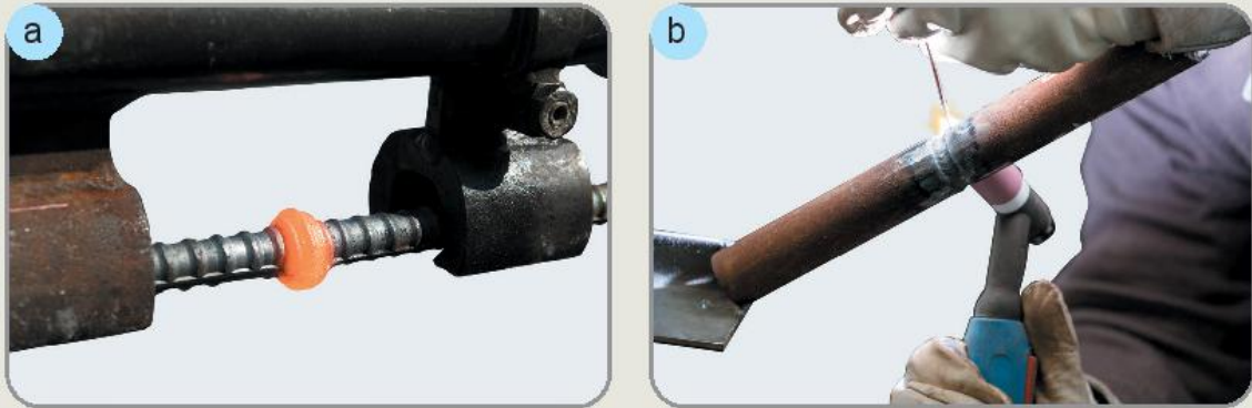
Hình 3.6. Chi tiết hàn
