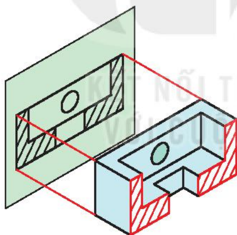
a) Chiếu phần vật thể còn lại
