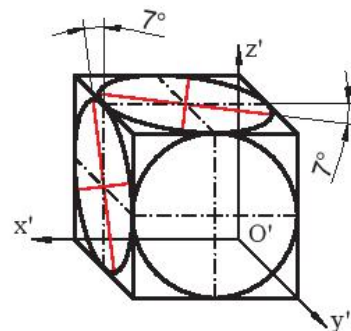
Hình 11.11. Các elip trong HCTĐ xiên góc cân
