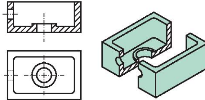
Hình 10.6. Hình cắt toàn bộ
