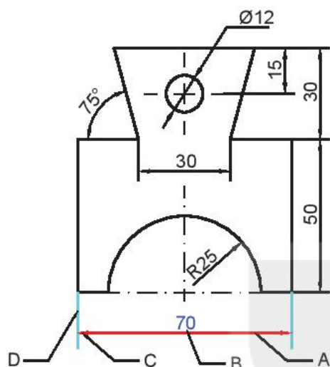
Hình 8.9. Giá đỡ
