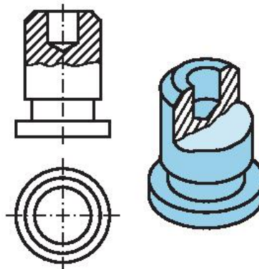
Hình 10.8. Hình cắt cục bộ
