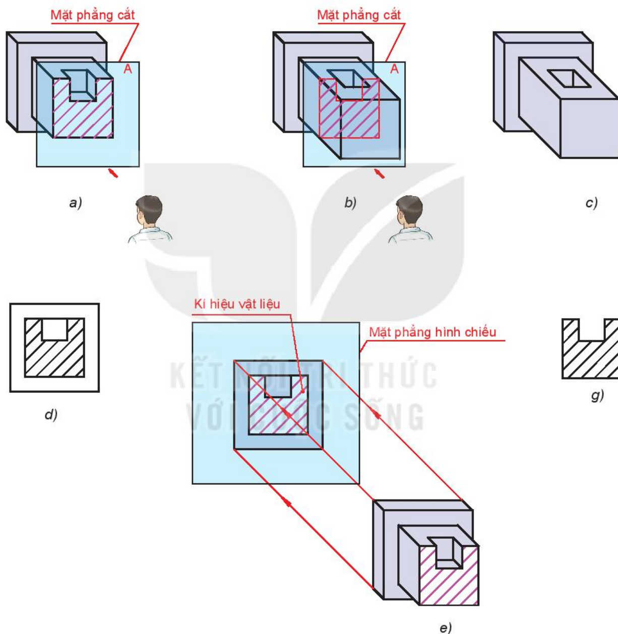
Hình 10.2. Sự hình thành mặt cắt, hình cắt
