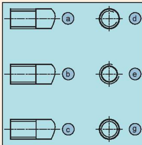
Hình 13.8. Ren trục
