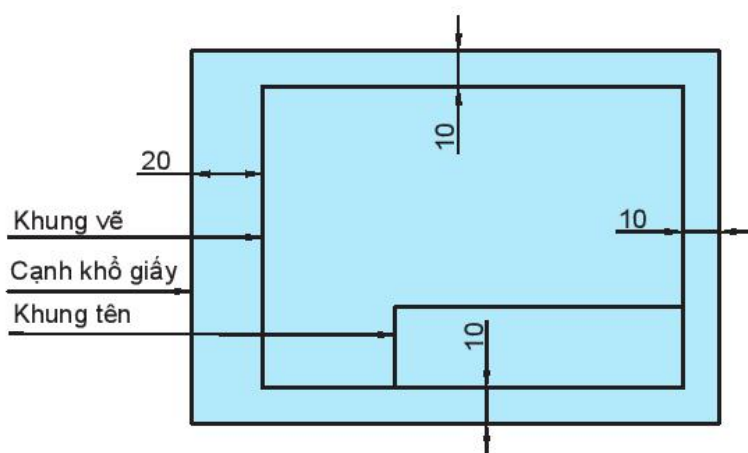
Hình 8.5. Khung bản vẽ và khung tên
