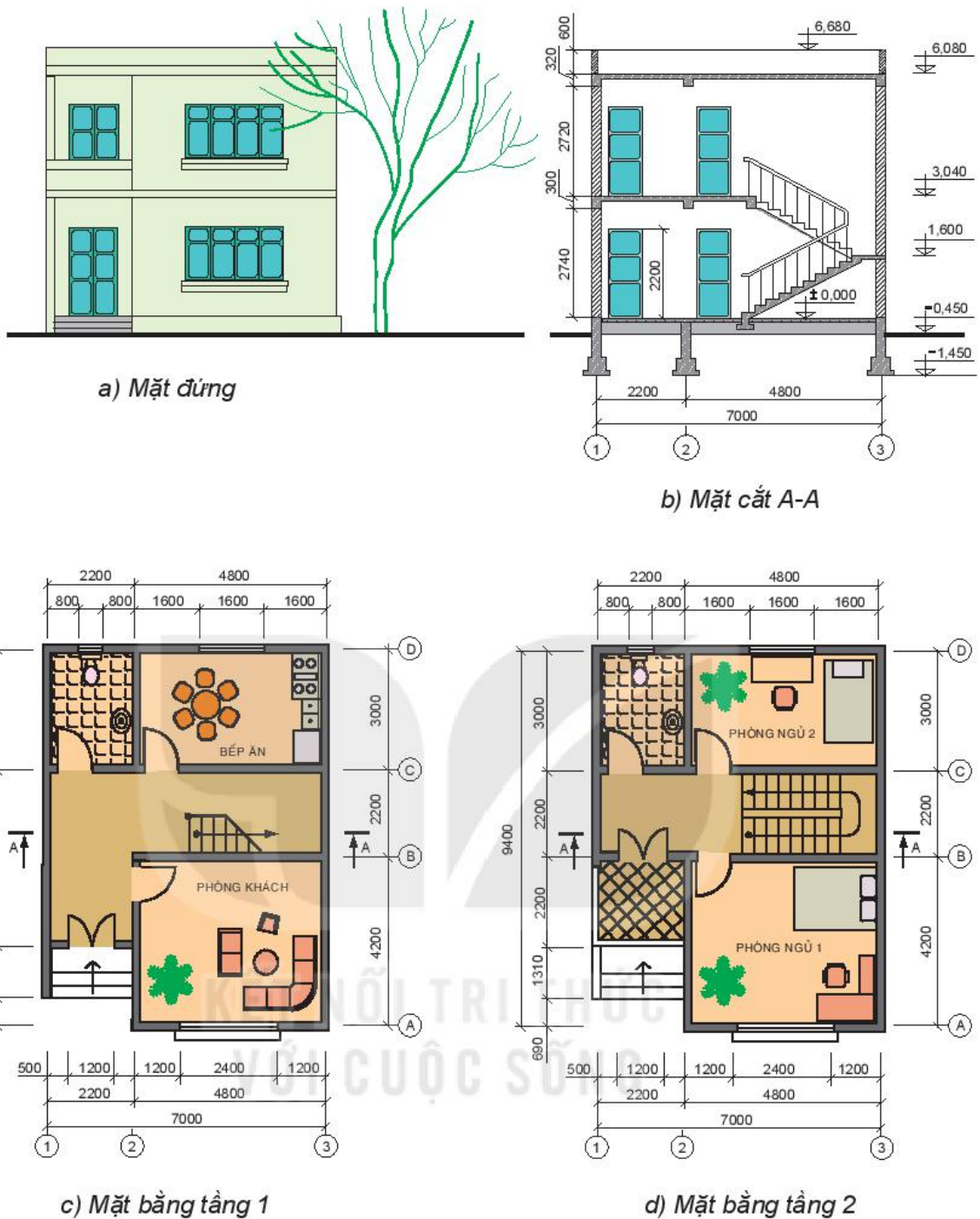
Hình 15.3. Bản vẽ nhà hai tầng
