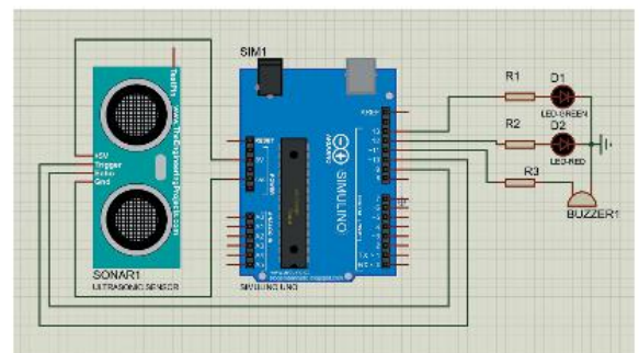
c) Thiết kế mạch điện tử
