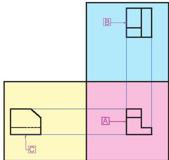
Hình 9.8. Các hình chiếu vuông góc
