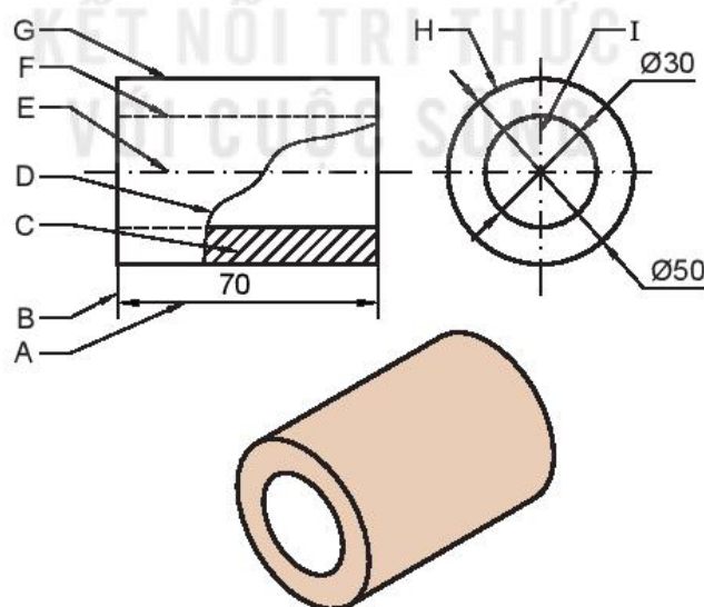
Hình 8.7. Bạc đỡ
