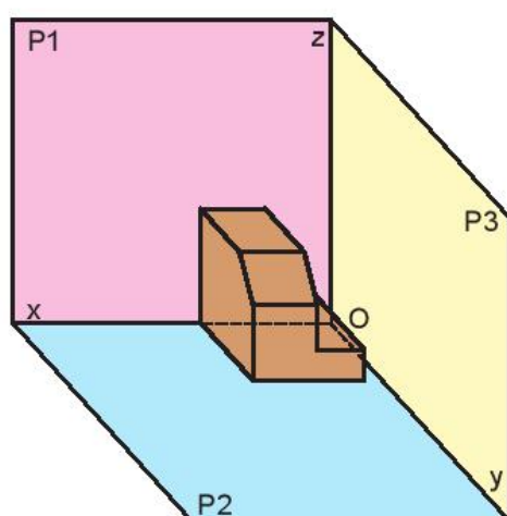
Hình 9.2. Các mặt phẳng hình chiếu
