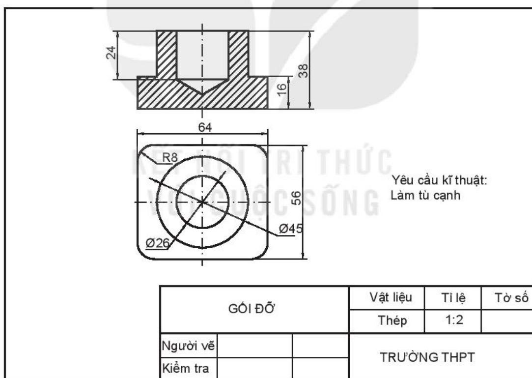
Hình 14.2. Bản vẽ gối đỡ
