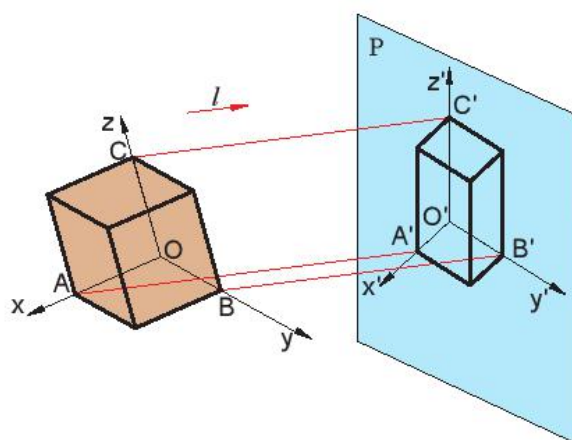
Hình 11.2. Xây dựng hình chiếu trực đo
