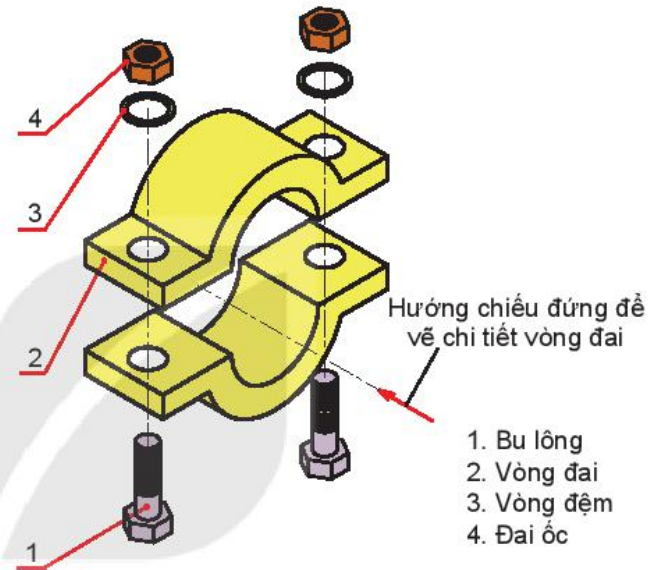
Hình 14.3. Cấu tạo bộ vòng đai
