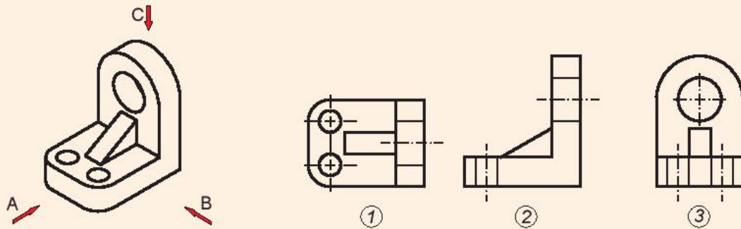
Hình 9.9. Gối đỡ
