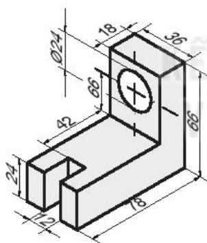
Hình 9.10. Giá đỡ
