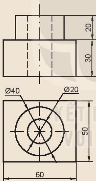
Hình 11.18. Gối đỡ
