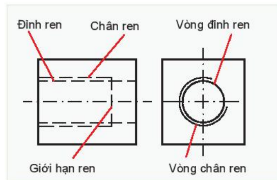
Hình 13.7. Ren khuất
