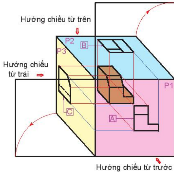
Hình 9.7. Phương pháp chiếu góc thứ ba
