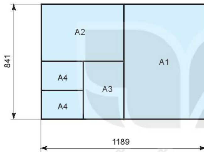
Hình 8.4. Các khổ giấy chính
