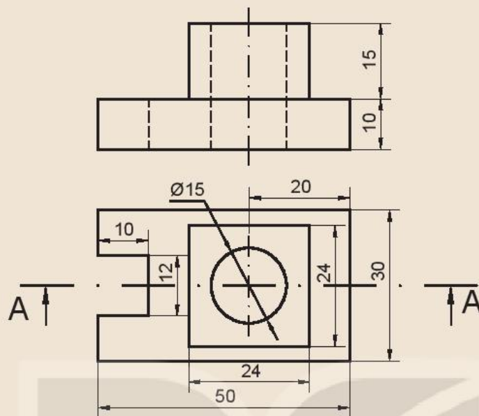
Hình 10.16. Đế
