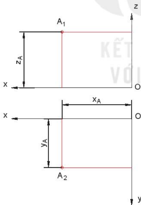
a) Hình chiếu vuông góc
