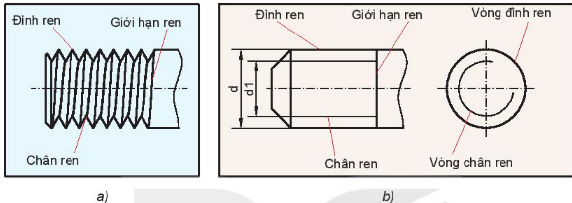
Hình 13.5. Biểu diễn ren ngoài
