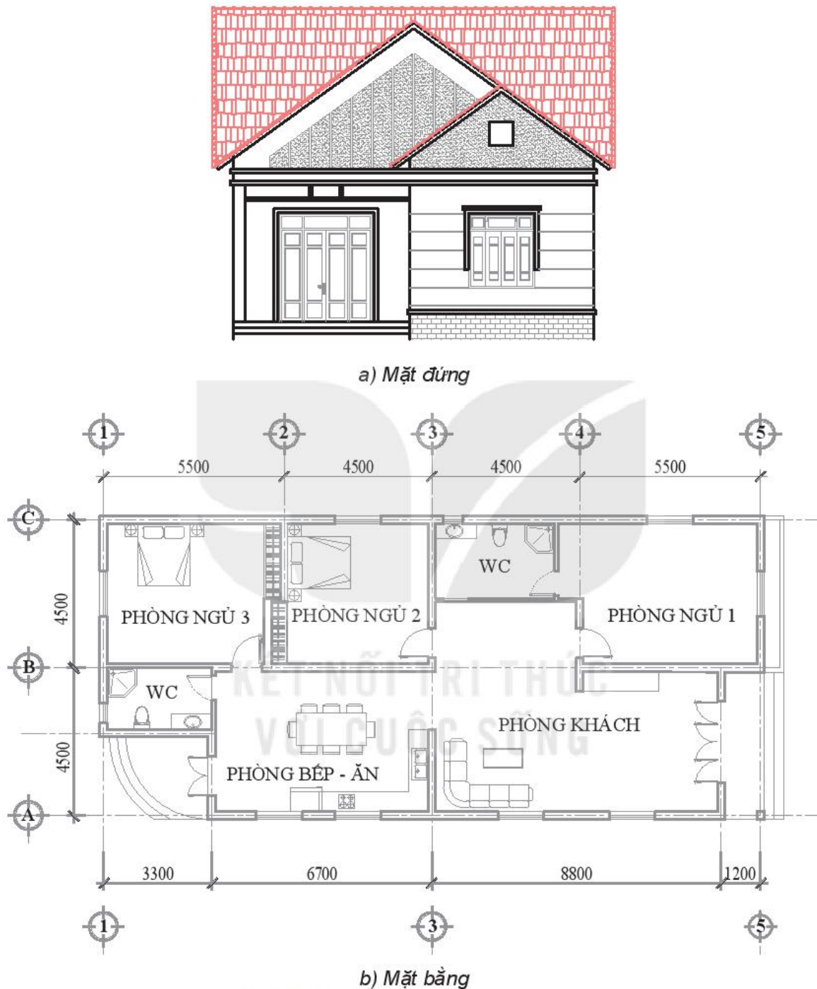
Hình 15.4. Bản vẽ ngôi nhà một tầng
