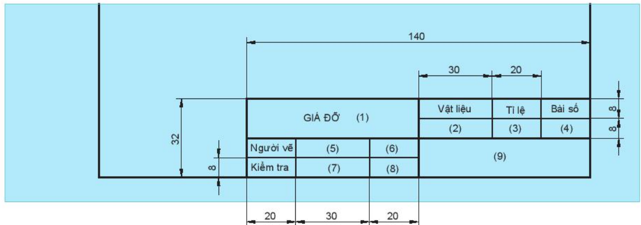
Hình 8.6. Kích thước và nội dung khung tên
