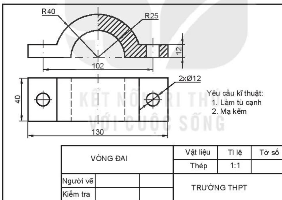
Hình 14.7. Bản vẽ chi tiết vòng đai
