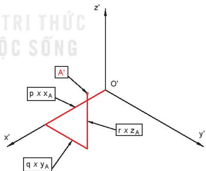
b) Hình chiếu trục đo
