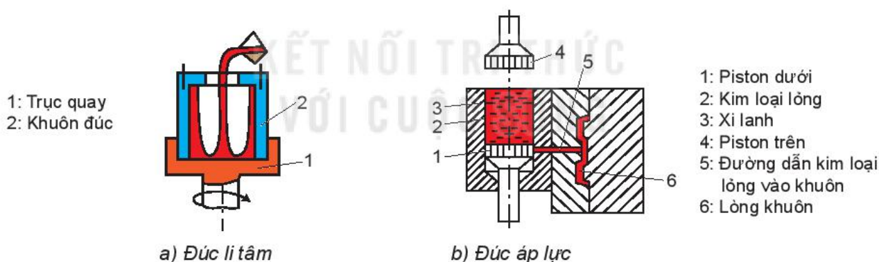
Hình 3.3. Một số công nghệ đúc
