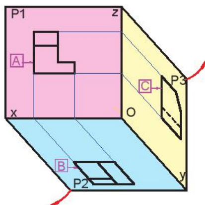
Hình 9.4. Quay các mặt phẳng hình chiếu
