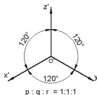
Hình 11.5. Góc trực đo và hệ số biến dạng
