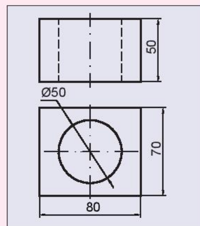
Hình 8.11. Giá đỡ
