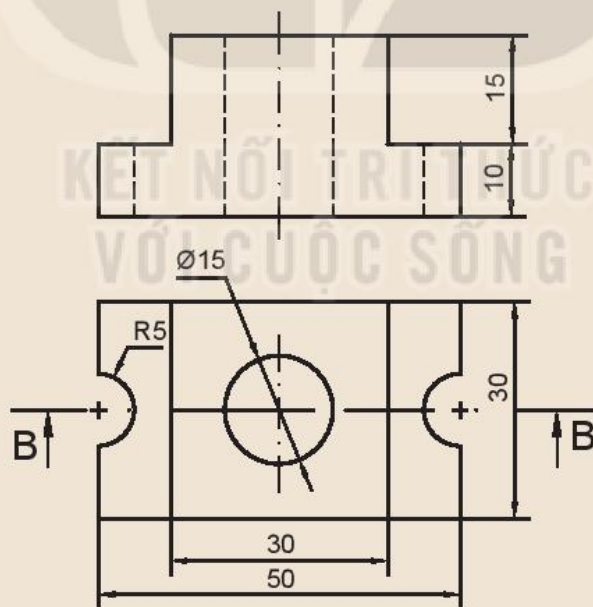
Hình 10.17. Gối đỡ
