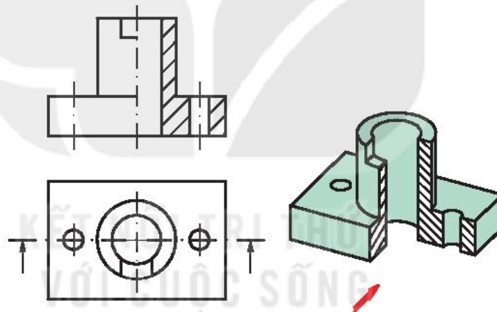
Hình 10.7. Hình cắt một nửa
