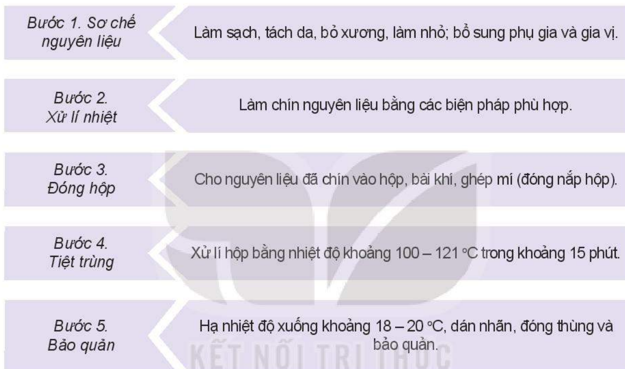
Hình 20.6. Sơ đồ các bước sản xuất thịt hộp
