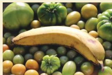
Hình 16.7. Khí ethylene sinh ra từ chuối sẽ làm cà chua xanh mau chín
