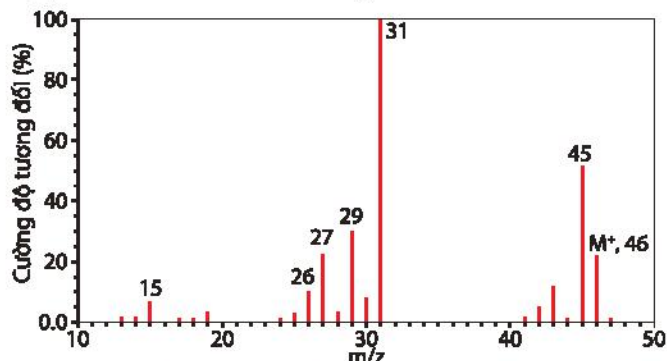
Hình 12.1. Phổ khối lượng của ethanol ( \text{C}_2\text{H}_6\text{O} ) (1)
