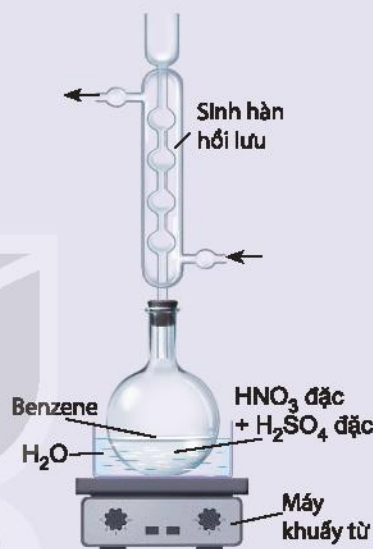
Hình 17.2. Thí nghiệm nitro hoá benzene
