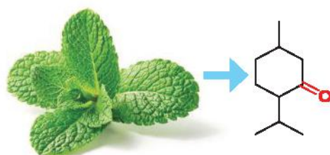
Hình 23.2. Menthone là một hợp chất ketone có trong tinh dầu bạc hà
