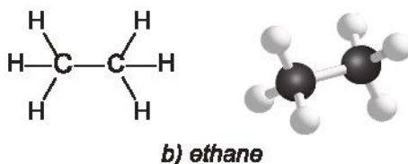
Hình 15.1. Công thức cấu tạo và mô hình phân tử của methane và ethane
