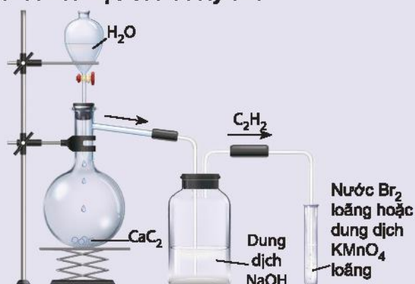
Hình 16.6. Điều chế acetylene và thử tính chất
