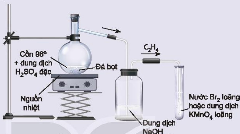
Hình 16.5. Điều chế ethylene và thử tính chất
