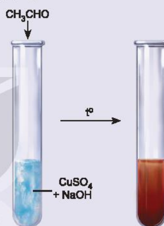
Hình 23.5. Phản ứng của \text{CH}_3\text{CHO} với \text{CuSO}_4 trong dung dịch \text{NaOH}
