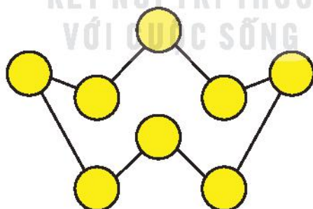
Hình 7.3. Phân tử sulfur \text{S}_8
