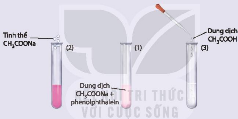
Hình 1.4. Ảnh hưởng của nồng độ đến sự chuyển dịch cân bằng
