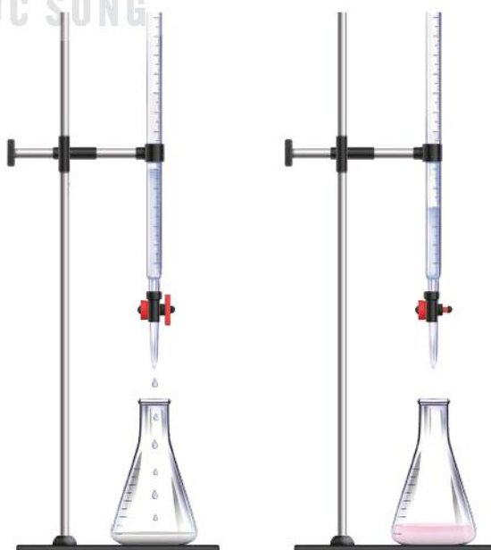
Hình 2.6. Chuẩn độ dung dịch NaOH bằng dung dịch HCl
