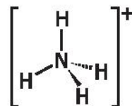
Hình 5.3. Dạng hình học của ion ammonium
