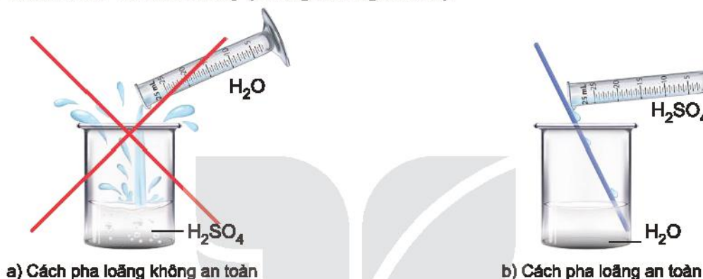
Hình 8.2. Cách pha loãng dung dịch sulfuric acid đặc
