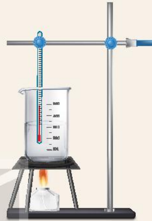
Hình 26.6 Bố trí thí nghiệm theo dõi nhiệt độ của nước khi đun sôi
