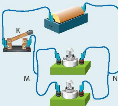
b) Hai bóng đèn mắc song song
