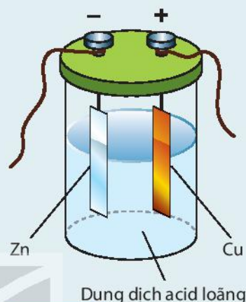
Hình 21.3 Cấu tạo pin Volta
