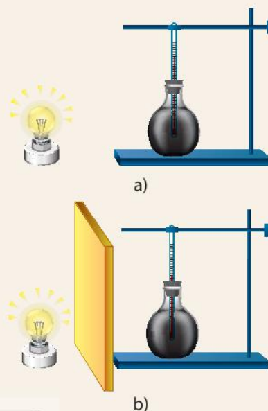
Hình 28.5 Bố trí thí nghiệm tìm hiểu bức xạ nhiệt
