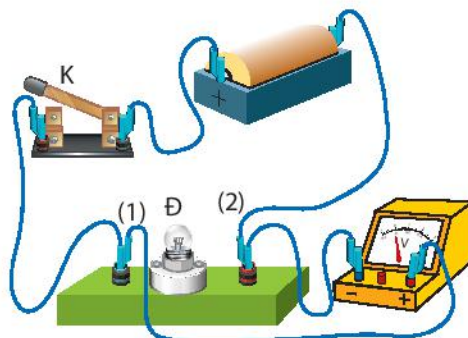
Hình 25.2 Mạch điện đo hiệu điện thế
