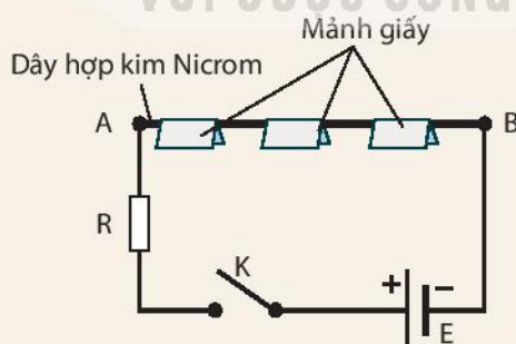
Hình 23.1 Sơ đồ mạch điện tìm hiểu về tác dụng nhiệt của dòng điện
