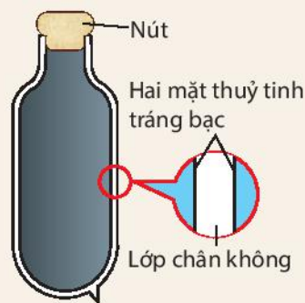
Hình 28.6 Cấu tạo ruột phích (bình thủy)
