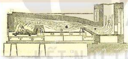
Hình 10. Lò luyện quặng theo phương pháp “pút-đinh” (Hen-ri Côt)
