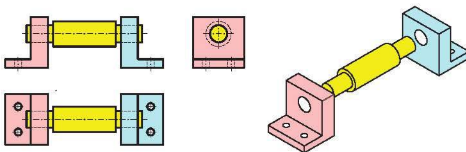
Hình 4.1. Tô màu chi tiết
