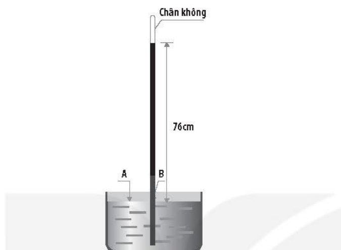
Hình 16.1. Thí nghiệm của Torricelli
