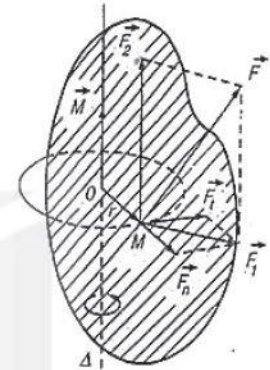
Hình 18.2. Tác dụng của lực trong chuyển động quay
