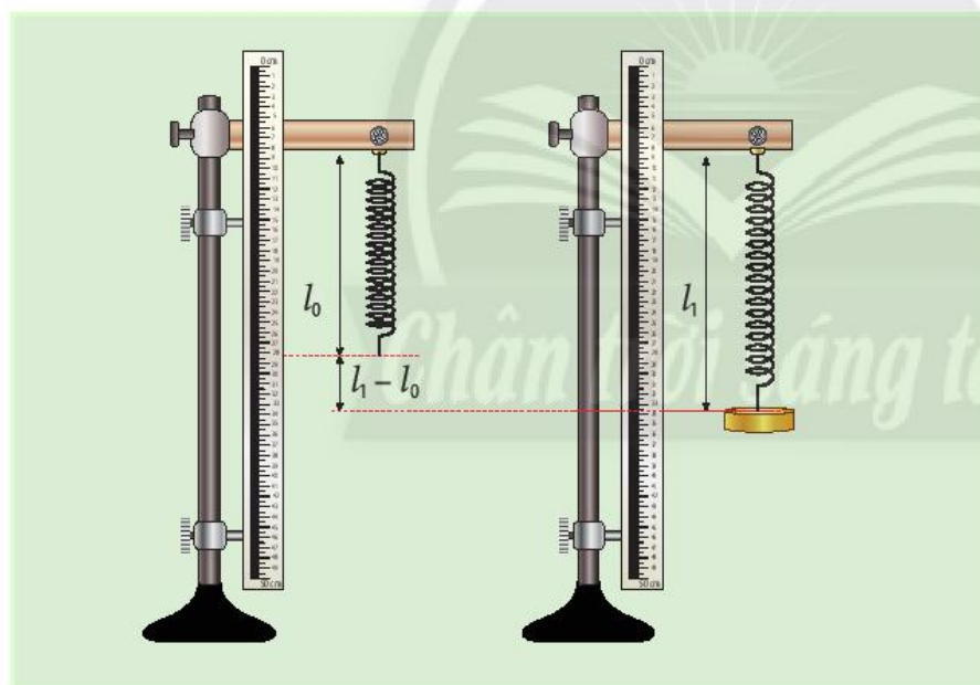
▲ Hình 39.1. Treo vật nặng vào lò xo
