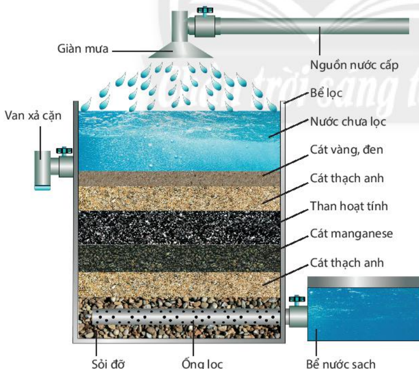
▲ Hình 16.1. Hệ thống lọc nước giếng bị nhiễm phèn
