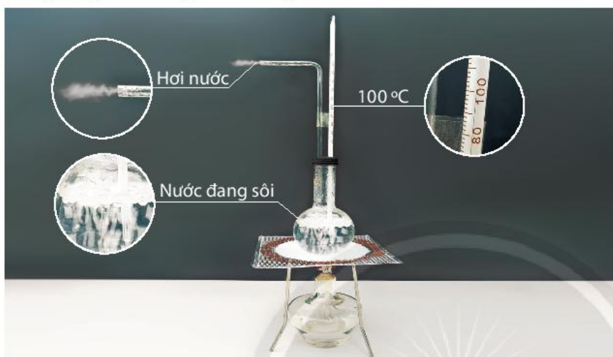
▲ Hình 8.7. Đo nhiệt độ sôi của nước
