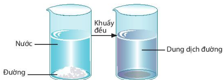
▲ Hình 15.11. Dung dịch
