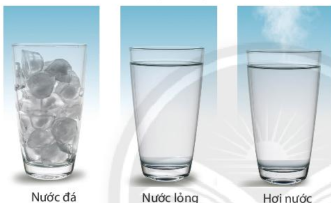
▲ Hình 8.2. Các thể của nước
