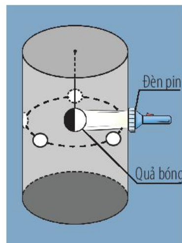
▲ Hình 44.6. Mô hình quan sát Mặt Trăng
