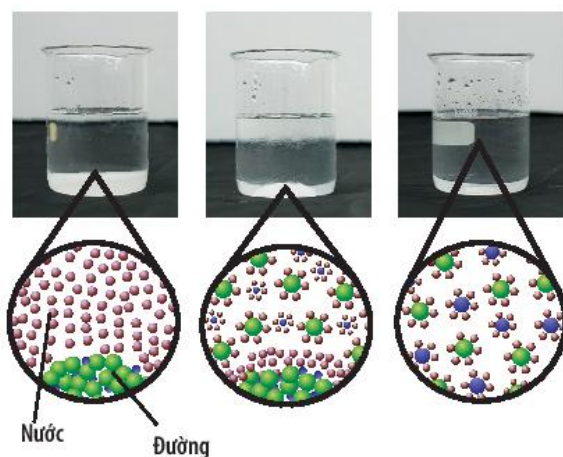
▲ Hình 15.8. Quá trình tạo dung dịch đường
