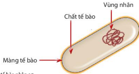
▲ Hình 17.4. Cấu tạo tế bào nhân sơ
