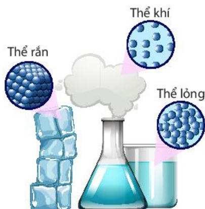
▲ Hình 8.3. Đặc điểm các thể của chất
