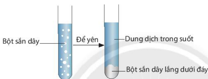
▲ Hình 15.12. Huyền phù
