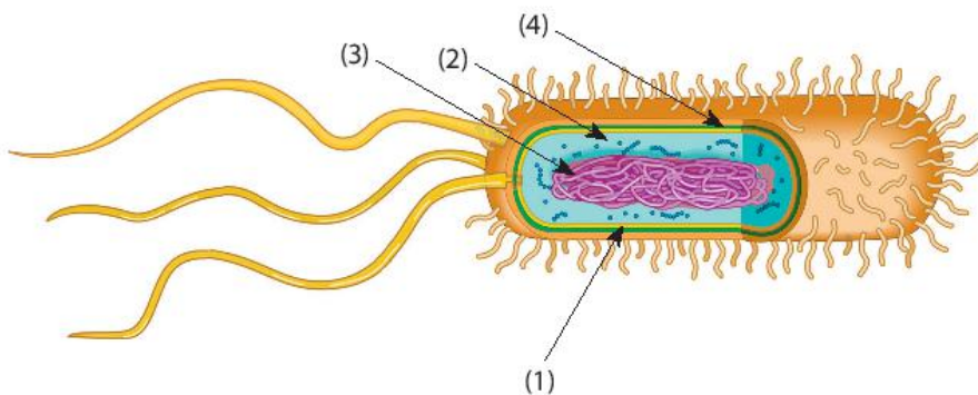
▲ Hình 25.2. Cấu tạo của vi khuẩn
