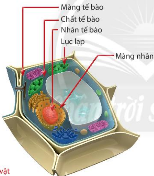
▲ Hình 17.5. Cấu tạo tế bào nhân thực
