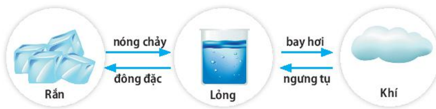
▲ Hình 8.17. Sự chuyển thể của chất
