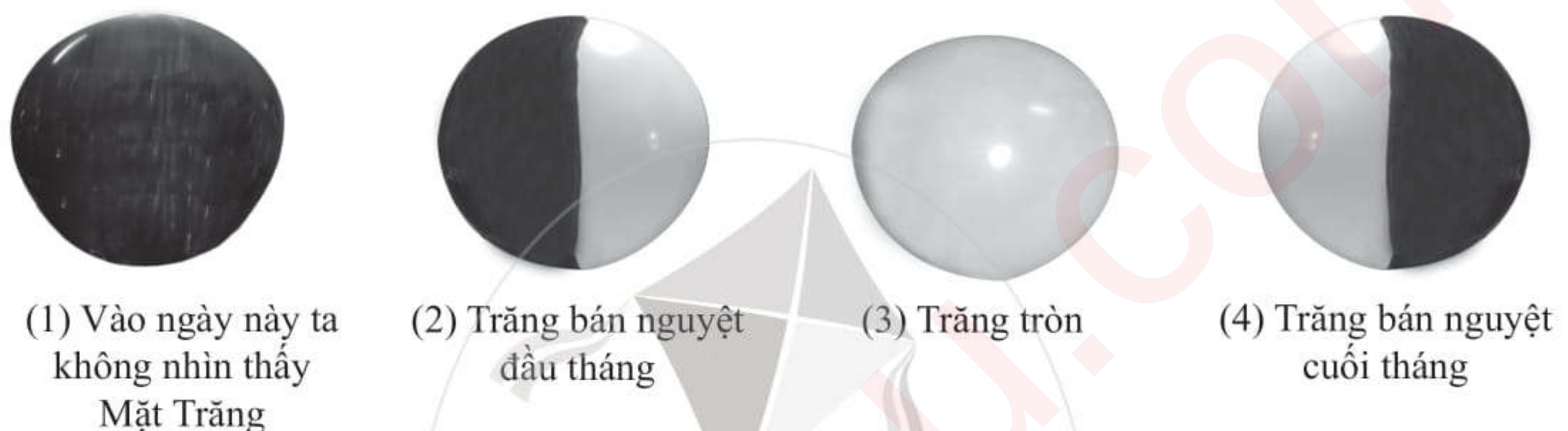
Hình 3. Các hình dạng cơ bản của Mặt Trăng tương ứng với các vị trí trên hình 2.
