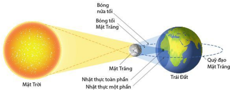
Hình 3.1. Sơ đồ giải thích nhật thực
