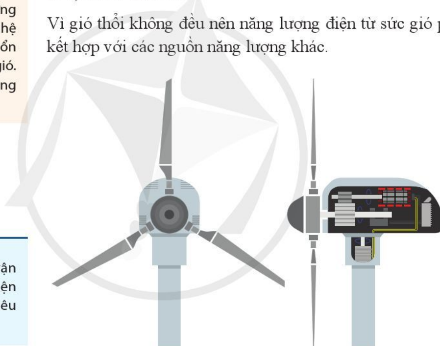
Hình 3.10. Cấu tạo của tua bin gió
