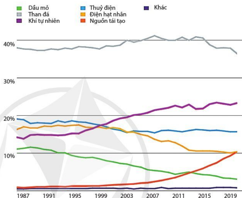
Hình 3.3. Sự thay đổi tỉ trọng năng lượng điện toàn cầu trong giai đoạn 1987 - 2019
