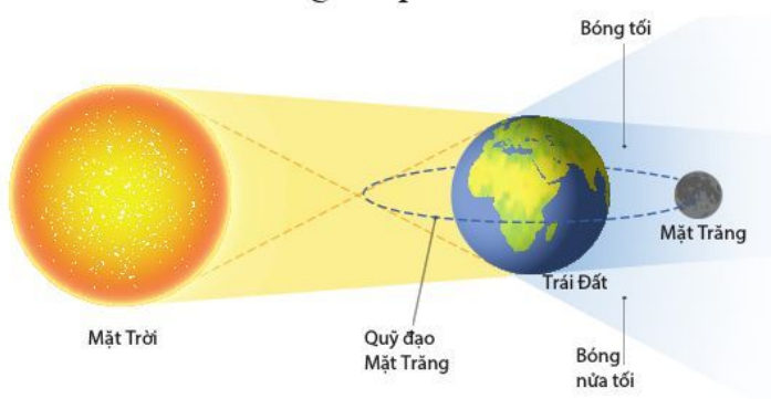
Hình 3.2. Sơ đồ giải thích nguyệt thực
