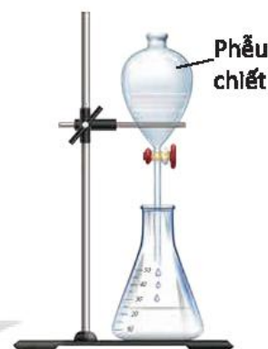
Hình 11.5. Dụng cụ chiết
