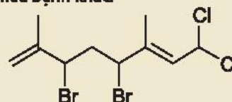
Hình 19.1. Dẫn xuất halogen tách ra từ tảo biển đỏ chỉ Laurencia có tác dụng chống ung thư vòm họng
