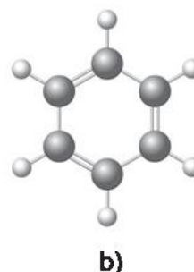
Hình 17.1. Công thức cấu tạo (a) và mô hình phân tử (b) của benzene
