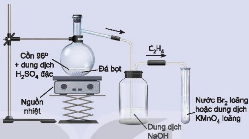
Hình 16.5. Điều chế ethylene và thử tính chất
